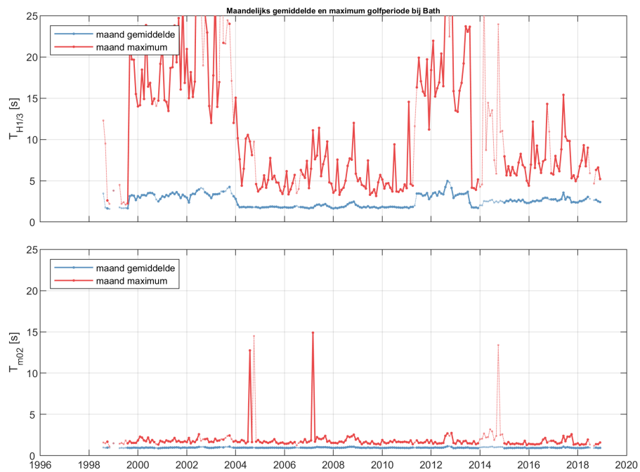
Figuur 2.52: Maandlijks gemiddelde en maximum van de golfperiode T_{H1/3} (boven) en T_{M02} (onder) voor station Bath.
