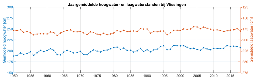
Figuur 2.8: Jaargemiddelde hoog- en laagwaterstanden bij Vlissingen
