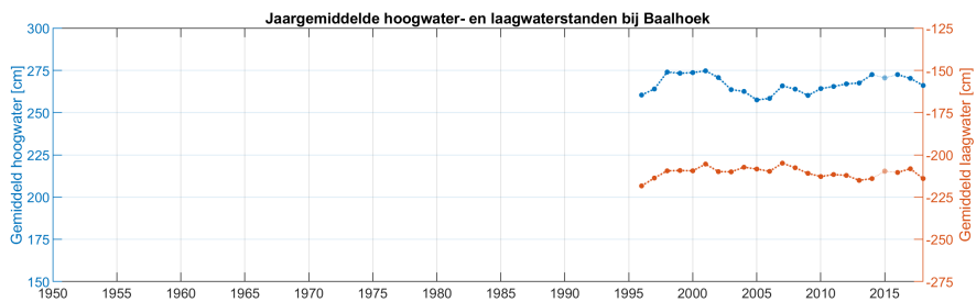
Figuur 2.14: Jaargemiddelde hoog- en laagwaterstanden bij Baalhoek
