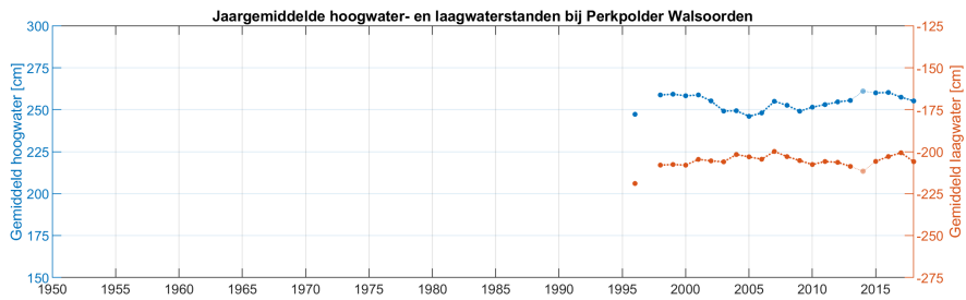
Figuur 2.13: Jaargemiddelde hoog- en laagwaterstanden bij Walsoorden
