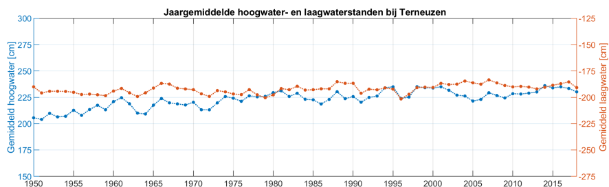
Figuur 2.11: Jaargemiddelde hoog- en laagwaterstanden bij Terneuzen
