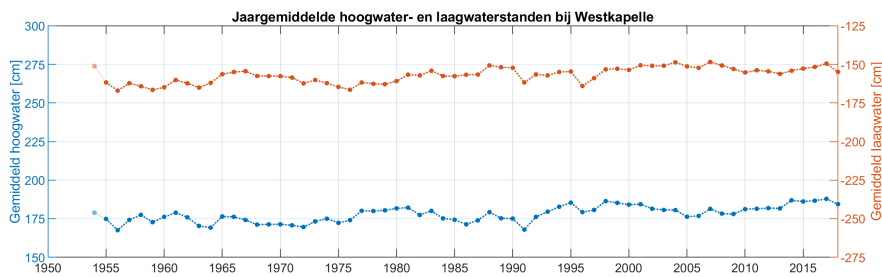
Figuur 2.6: Jaargemiddelde hoog- en laagwaterstanden bij Westkapelle
