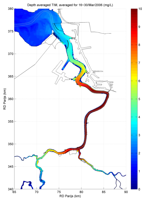
Figuur 4-14: Gemiddelde slibconcentratie (mg/l) over springtij – doottij cyclus bij eenheidslozing te Vliete van Hoboken.
