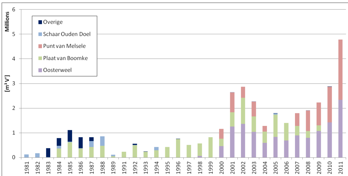
Figuur 2-2: Gebaggerde volumes slib in de Beneden-Zeeschelde opgesplitst naar bron (boven) en opgesplitst naar stortlocatie.
