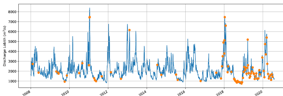
Figuur 3-1. Verloop van afvoer bij Lobith (blauw) met tijdstippen waarop de verhanglijnmetingen zijn uitgevoerd (oranje). Tot augustus 2017 zijn verhanglijnen alleen in de rivieras gemeten. Vanaf augustus 2017 zijn de metingen ook langs de linkeroever, langs de rechteroever en in de drie oevergeulen uitgevoerd.
