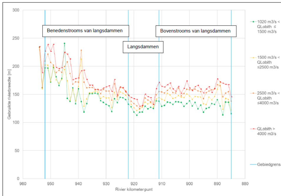
Figuur 7-2. Gebruikte rivierbreedte voor verschillende bereiken van de afvoer, gedefinieerd als de breedte waarbinnen 90% van de schepen vaart (Indah-Everts & Hermans, 2021).
