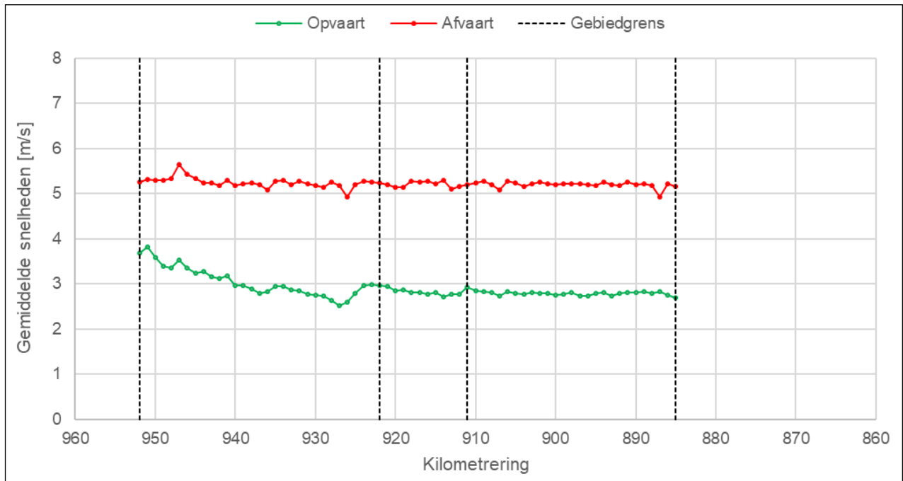
Figuur 3-28 Gemiddelde vaarsnelheid profiel voor schepen met diepgang > 3.5 m tussen januari 2018 tot mei 2020 tijdens 1500 \text{ m}^3/\text{s} < Q_{Lobith} \leq 2500 \text{ m}^3/\text{s}
