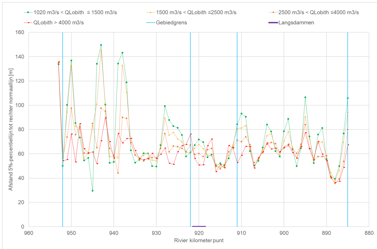
Figuur 3-25 Passeerafstand tot rechter normaallijn zowel opvaart als afvaart tijdens verschillende afvoerranges
