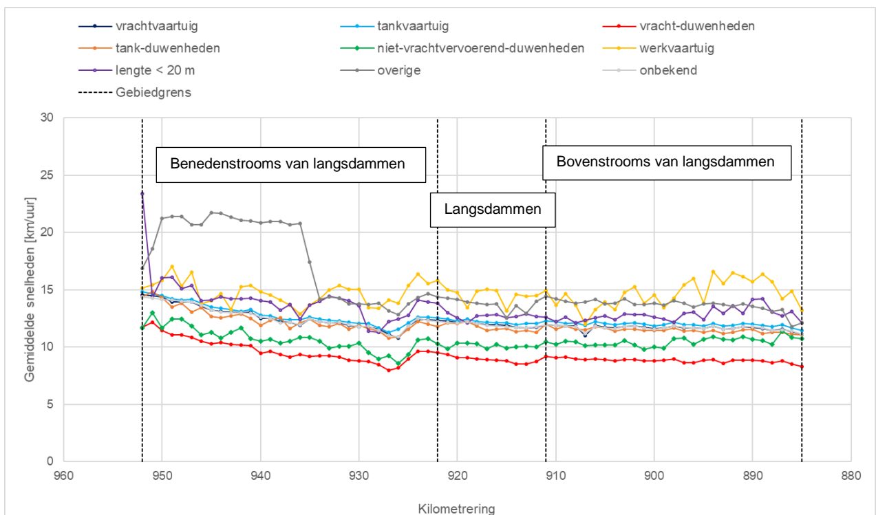
Figuur 3-7 Scheepssnelheid profiel langs het rivier – opvaart
