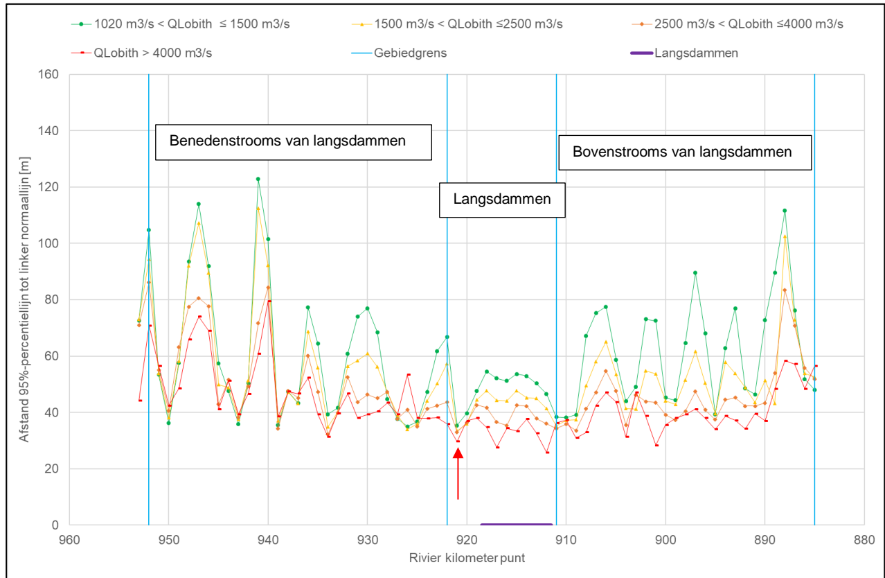
Figuur 3-22 Passeerafstand tot linker normaallijn zowel opvaart als afvaart tijdens verschillende afvoerranges
