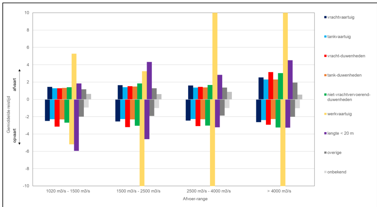
Figuur 3-1 Gemiddelde reistijd [uur] voor het bovenstrooms van langsdammen gebied [kmr 885 - 911] per richting per scheepstype per afvoerranges
