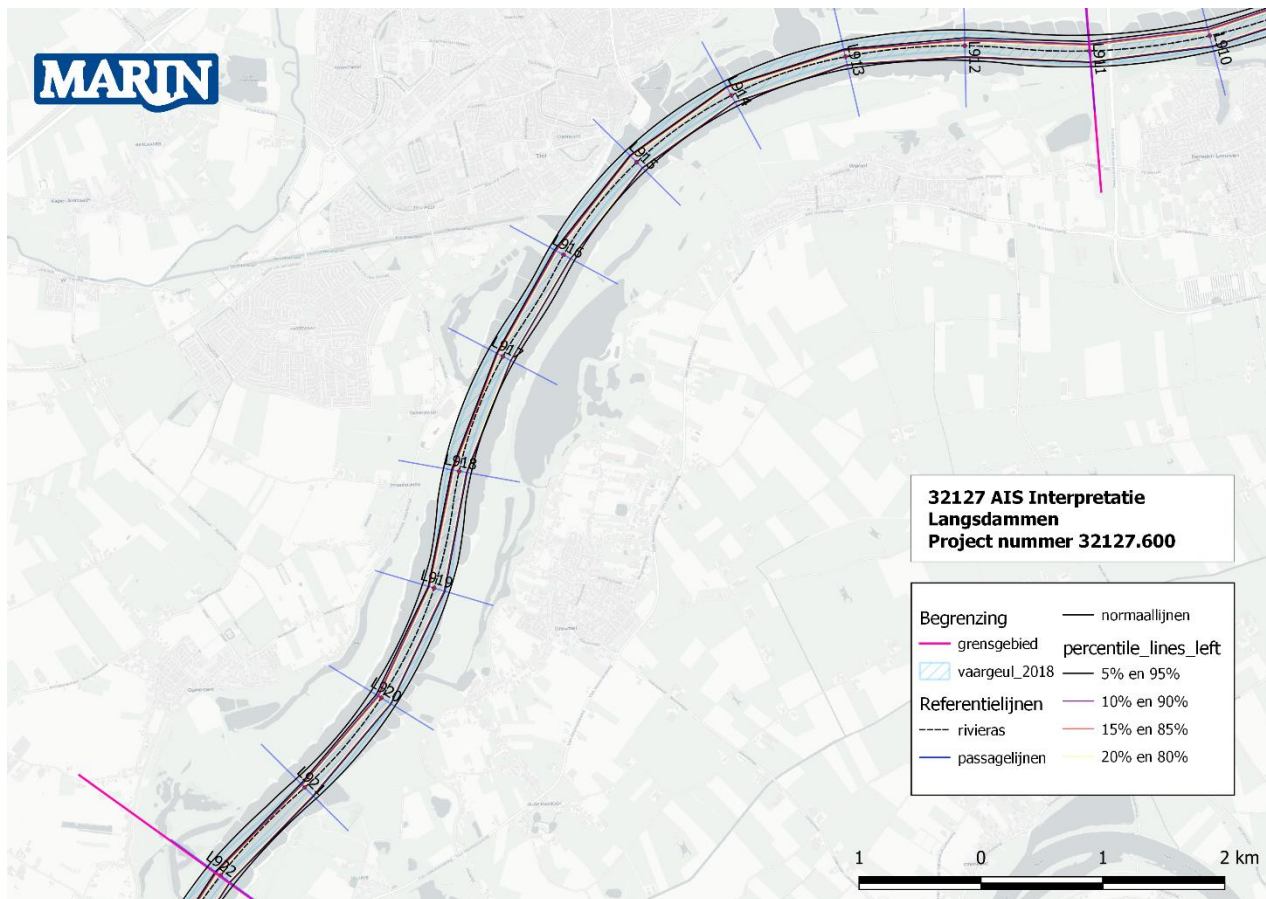
Figuur 3-12 Ruimtegebruik het langsdammen gebied [kvr 911 - 922] tijdens Q_{Lobith} > 4000 \text{ m}^3/\text{s}
