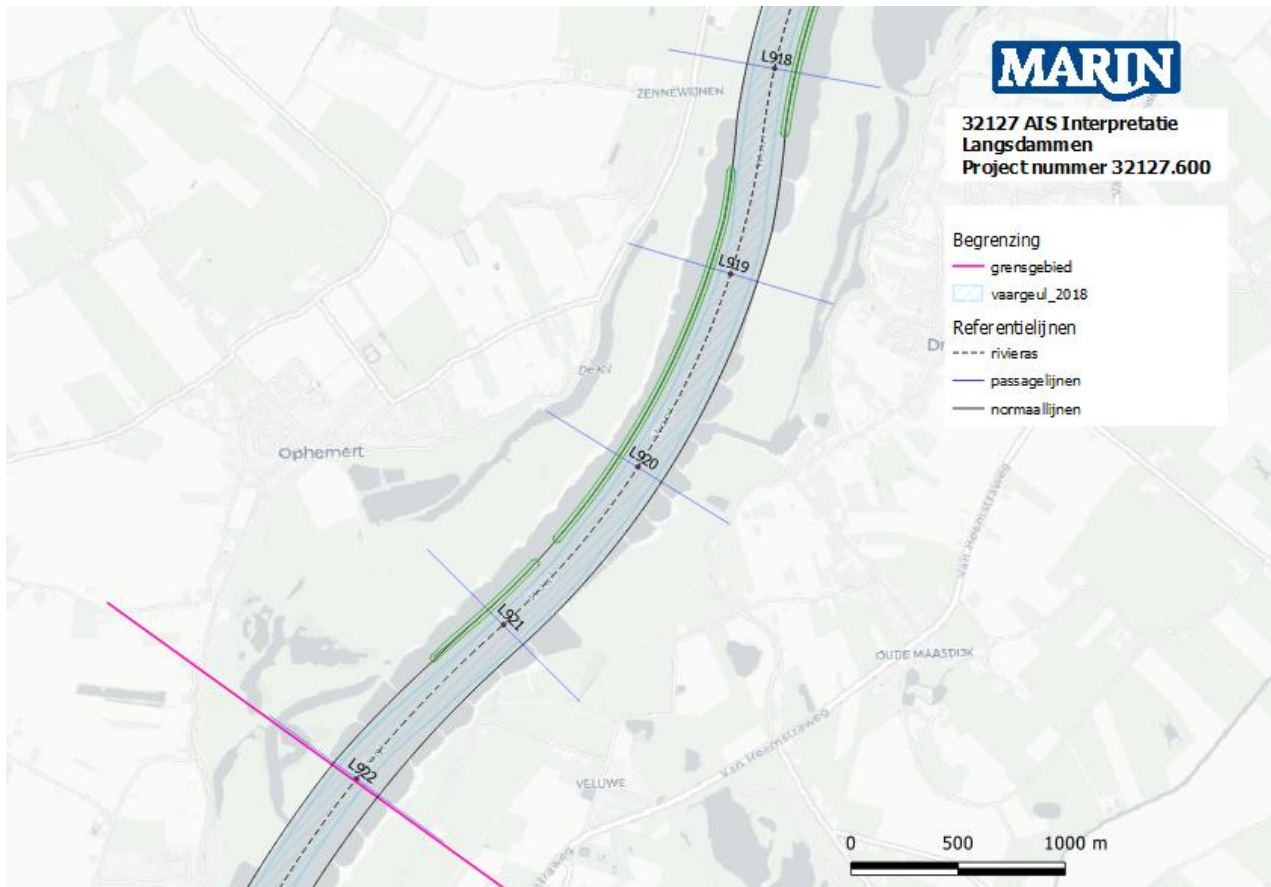
Figuur 3-24 Locatie langsdammen aan de rechter normaallijn
