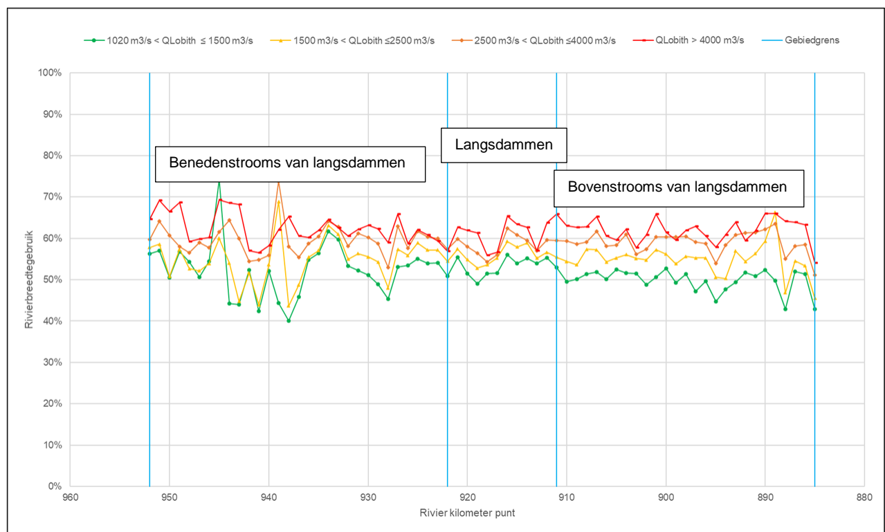
Figuur 3-19 Genormaliseerde rivierbreedtegebruik tijdens verschillende afvoerranges
