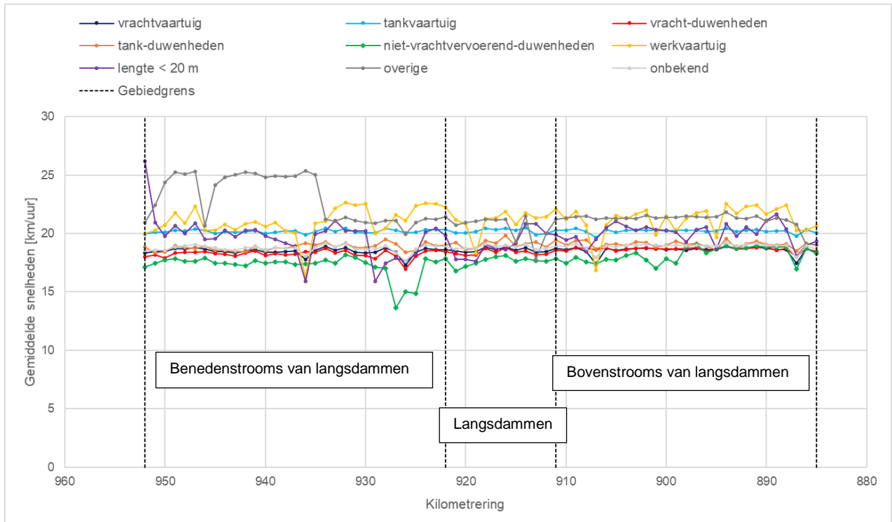
Figuur 3-6 Scheepssnelheid profiel langs het rivier - afvaart
