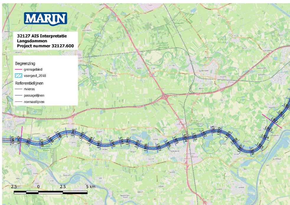
Figuur 2-4 Benedenstroomse langsdammen gebied
