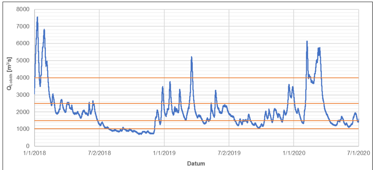
Figuur 2-8 Afvoer Lobith tussen januari 2018 tot juni 2020
