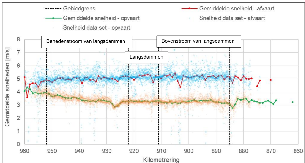
Figuur 3-27 Gemiddelde vaarsnelheid profiel voor schepen met diepgang > 3.5 m tussen 31 mei tot 10 juni 2012
