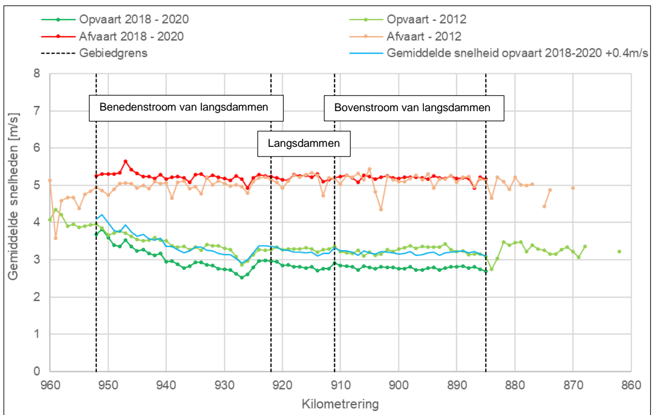
Figuur 3-29 Gemiddelde vaarsnelheid profiel voor schepen met diepgang > 3.5 m verschil 2012 met periode tussen januari 2018 tot mei 2020
