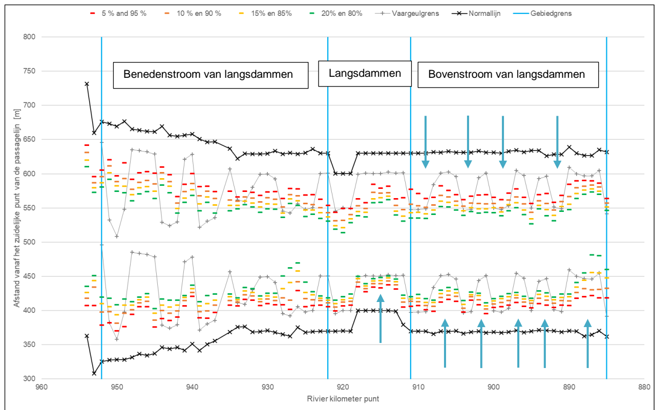
Figuur 3-16 Ruimtegebruik tijdens Q_{Lobith} > 4000 \text{ m}^3/\text{s}
