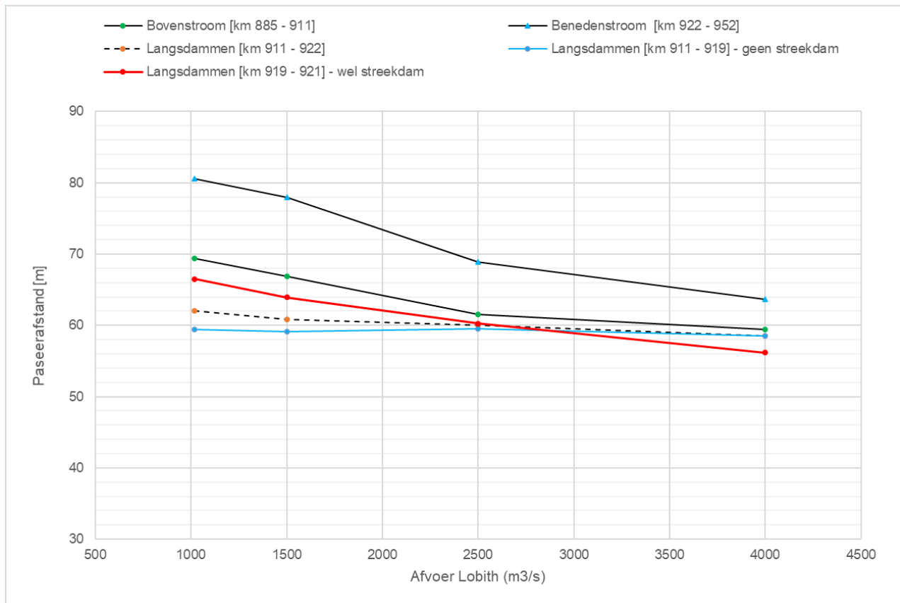
Figuur 3-26 Gemiddelde passeerafstand tot rechter normaallijn tijdens verschillende afvoerranges
