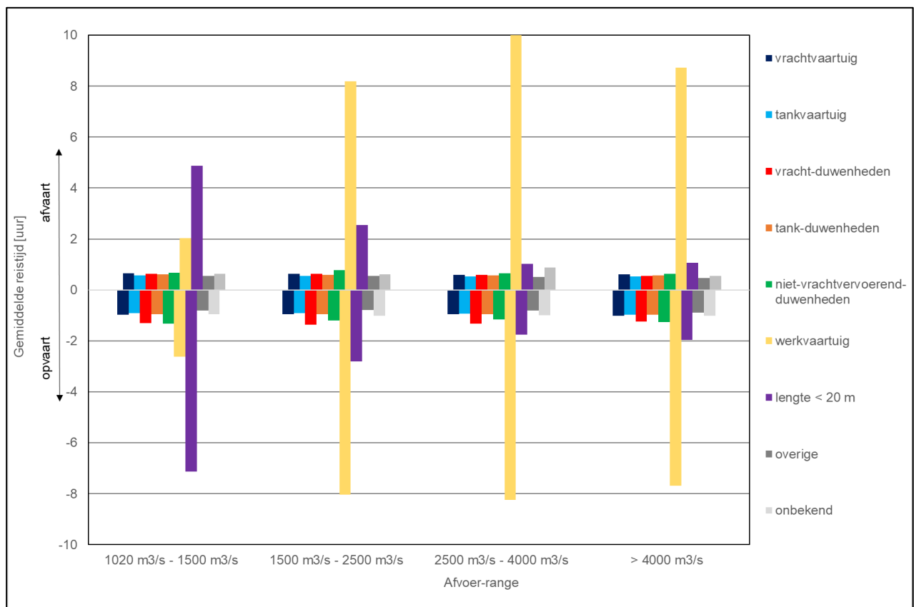
Figuur 3-2 Gemiddelde reistijd [uur] voor langsdammen gebied [kvr 911 - 922] per richting per scheepstype per afvoerranges
