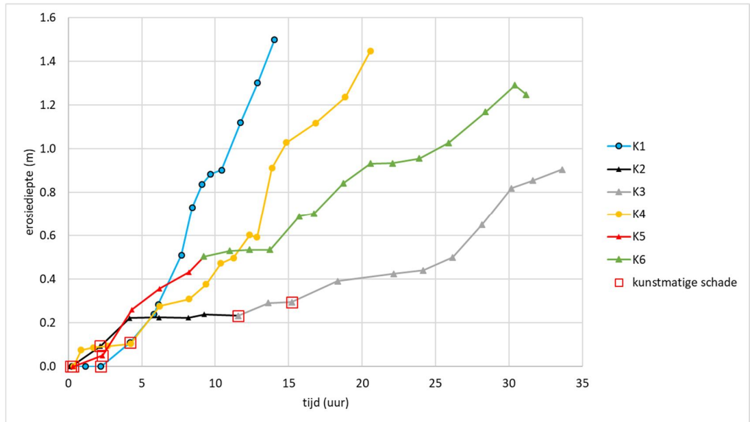
Fig. E-1 Gemeten erosiediepte als functie van de tijd van alle Deltagootproeven
