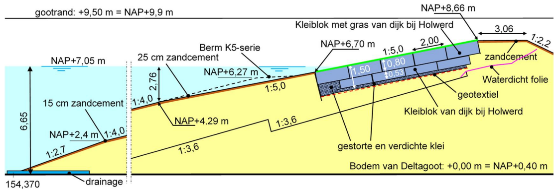
Figuur 3.22 Modelopstelling voor proevenserie K6
