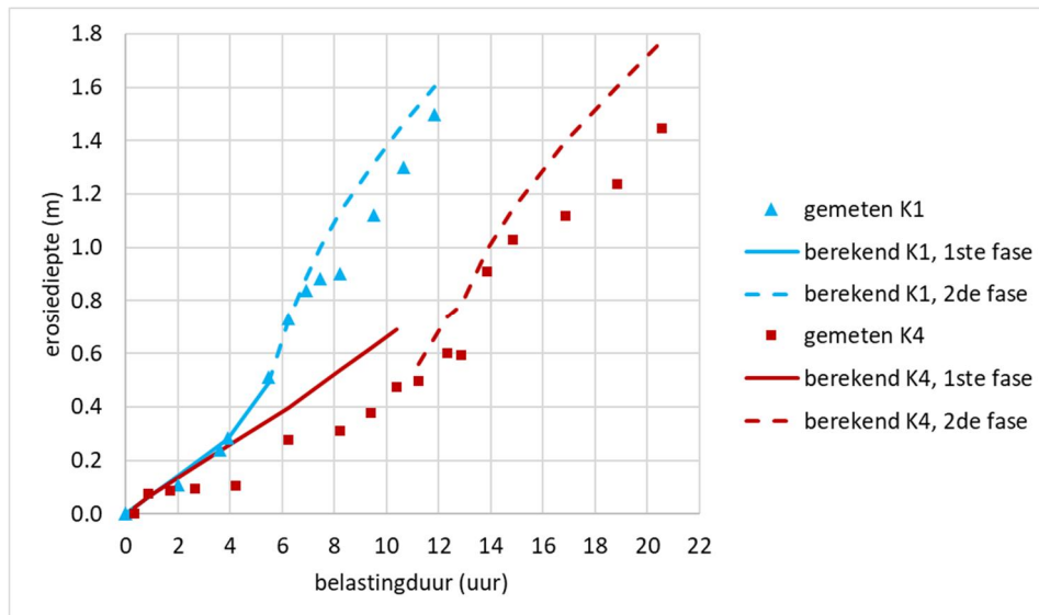
Figuur 5.29 Berekende erosiediepte en gemeten waarde in de Deltagoot van serie K1 en K4 (talud 1:4 met klei van de Lauwersmeerdijk en Blija)
