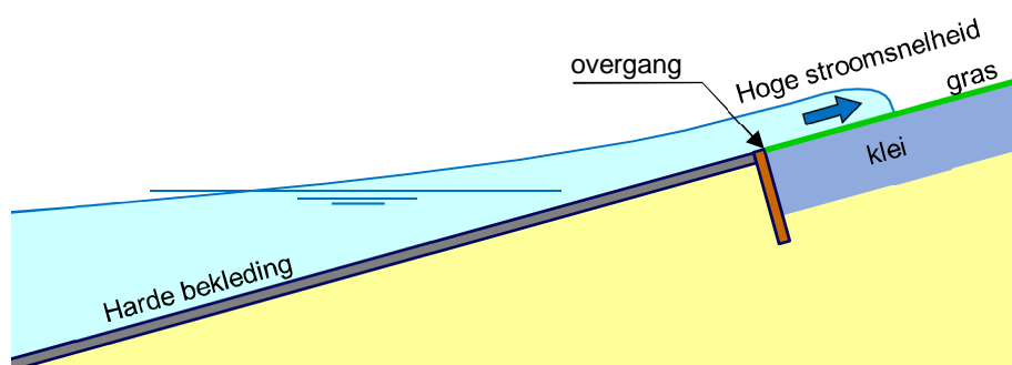
Figuur 4.1 Belasting door golfloop: hoge stroomsnelheid over het gras
