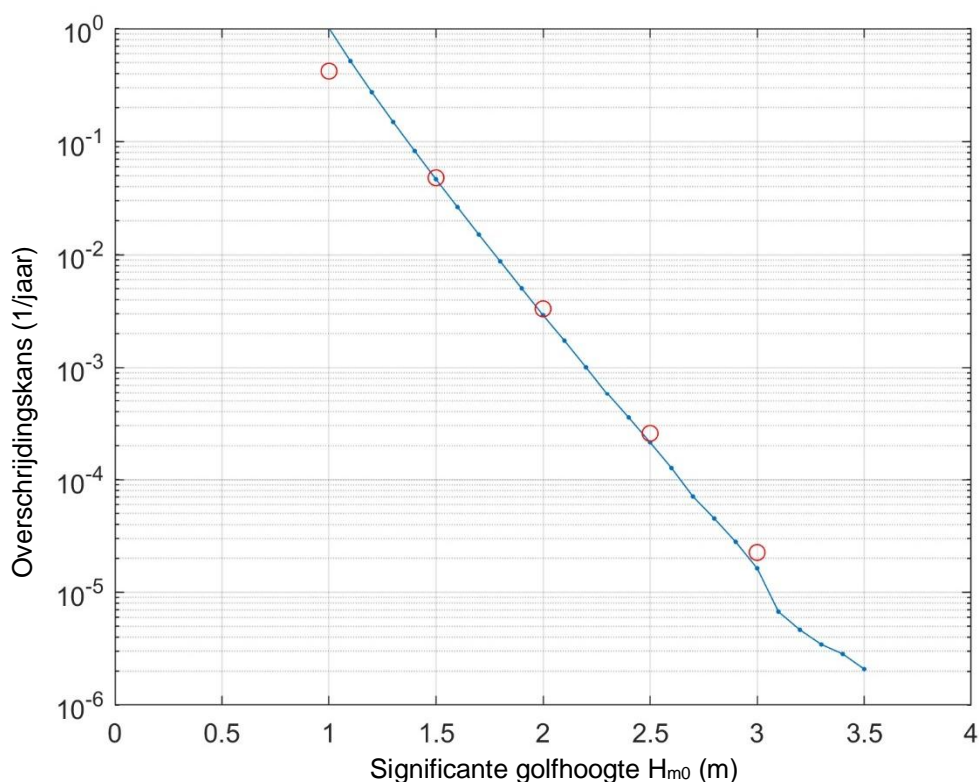
Figuur 7.4 Overschrijdingskromme van de significante golfhoogte op basis van Hydra-NL (rode rondjes) en punten uit de beschouwde golfcondities in de Monte Carlo simulatie voor het jaar 2075 (blauwe lijn) voor locatie 3
