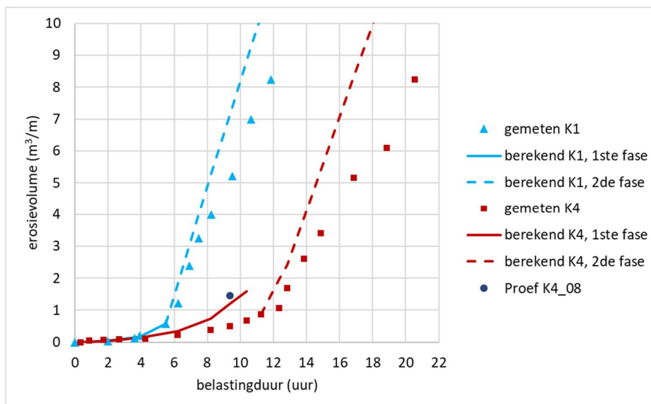
Figuur 5.30 Berekende erosievolume en gemeten waarde in de Deltagoot van serie K1 en K4 (talud 1:4 met klei van de Lauwersmeerdijk en Blija)
