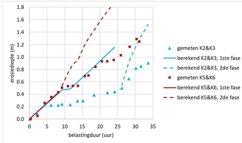
Figuur 5.31 Berekende erosiediepte en gemeten waarde in de Deltagoot van serie K2&K3 en K5&K6 (talud 1:5 met klei van Holwerd)
