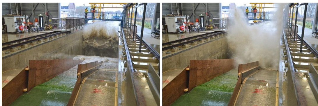
Figuur 8.3 Aanstormende golf en resulterende golfklap tijdens proef K5_03
