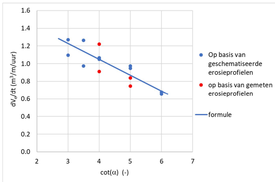
Figuur 5.27 Invloed van de taludhelling op de erosiesnelheid (de Deltagootproeven hadden een waarde van \cot\alpha = 4 en 5 )
