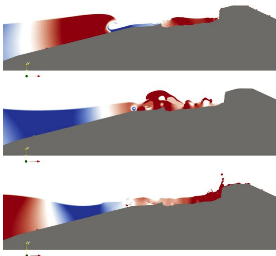
Figuur 5.12 Drie momenten tijdens het breken van een golf op de dijk met een erosiekuil op het boventalud.
