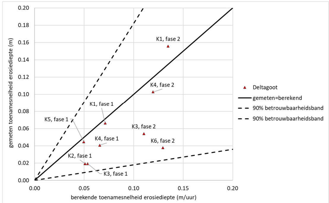
Figuur 5.33 In de Deltagoot gemeten gemiddelde erosiesnelheid als functie van de met de formules berekende erosiesnelheid (toename van de erosiediepte per uur)
