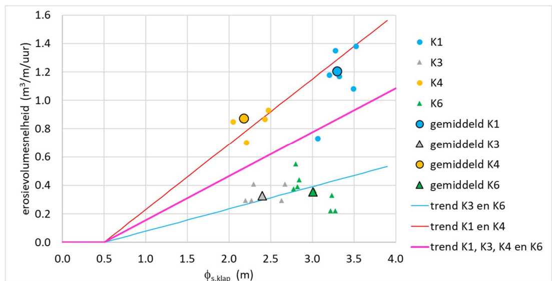
Fig. D-1 Relatie tussen berekende piekdruk uit OpenFoam ( \phi_{s,klap} ) en de gemeten erosiesnelheid ( \partial V_e/\partial t )
