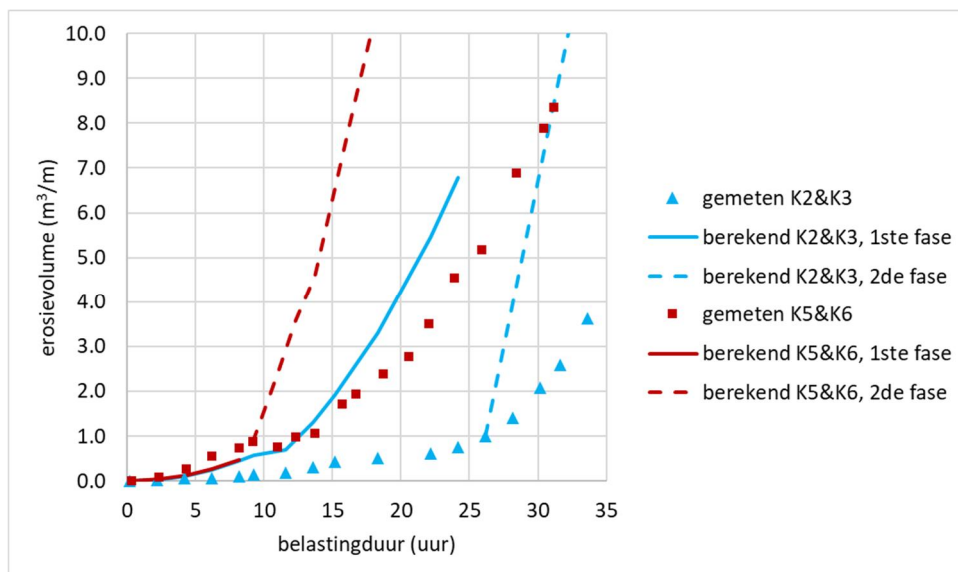
Figuur 5.32 Berekende erosievolume en gemeten waarde in de Deltagoot van serie K2&K3 en K5&K6 (talud 1:5 met klei van Holwerd)
