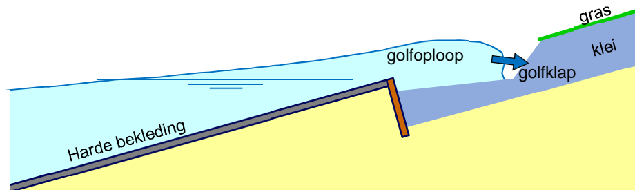
Figuur 4.4 Golfploop zorgt voor een golfklap tegen de klif
