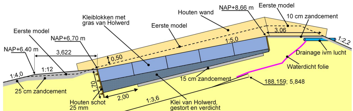
Figuur 3.9 Modelopstelling voor de tweede serie proeven (K2)
