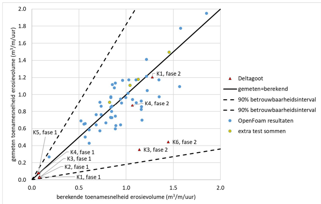
Figuur 5.34 In de Deltagoot gemeten gemiddelde erosiesnelheid en met OpenFoam berekende erosiesnelheid als functie van de met de formules berekende erosiesnelheid (toename van de erosievolume per uur)
