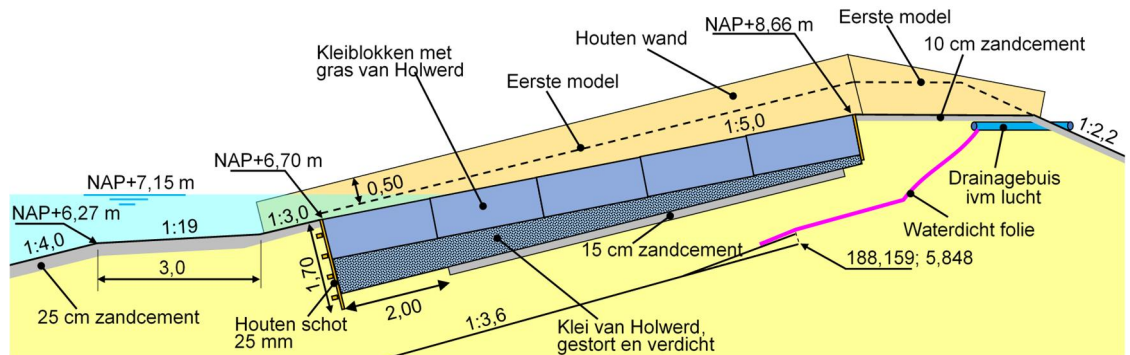
Figuur 3.10 Modelopstelling voor derde serie proeven (K3)
