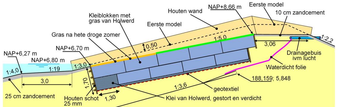
Figuur 3.21 Modelopstelling van proevenserie K5
