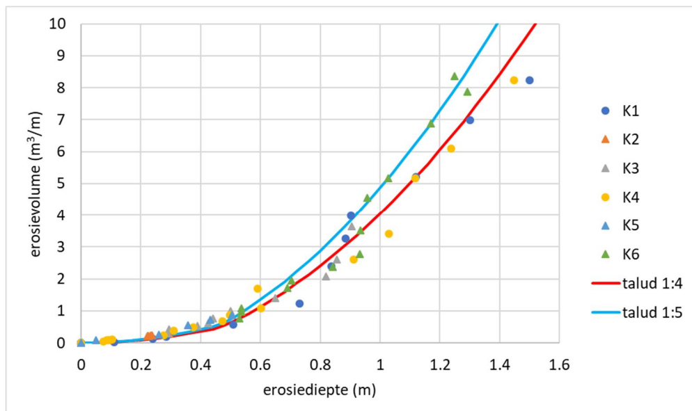
Figuur 5.4 Gemeten relatie tussen de erosiediepte en het erosievolume en de berekende relatie op basis van \tan\alpha_{\text{terras}} = 1/8 en \tan\alpha_{\text{klif}} = 2 voor een talud van 1:4 en \tan\alpha_{\text{terras}} = 1/10 en \tan\alpha_{\text{klif}} = 2 voor een talud van 1:5.
