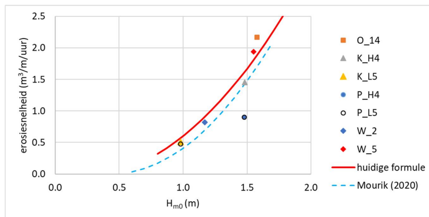
Figuur 5.28 De huidige formule in vergelijking tot die van Mourik (2020) en Deltagootmetingen die Mourik gebruikt heeft voor het afleiden van zijn formule
