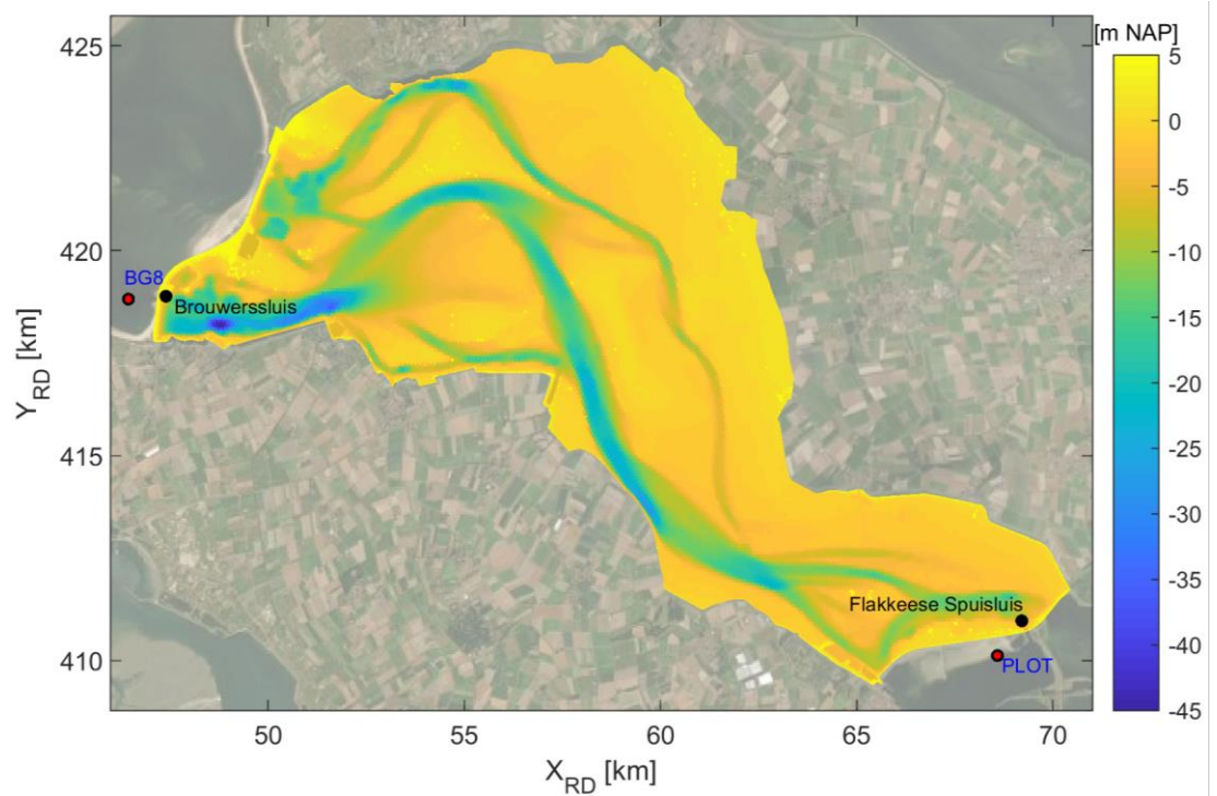
Figuur 4-13 Kunstwerken Brouwerssluis en Flakkeese Spuisluis. Saliniteit- en temperatuurgegevens van Brouwershavensche Gat 08 (BG8) en Plaat van Oude Tonge (PLOT) zijn gebruikt als randvoorwaarden ter plaatse van deze kunstwerken. In de achtergrond is de bodemligging in m NAP weergegeven.
