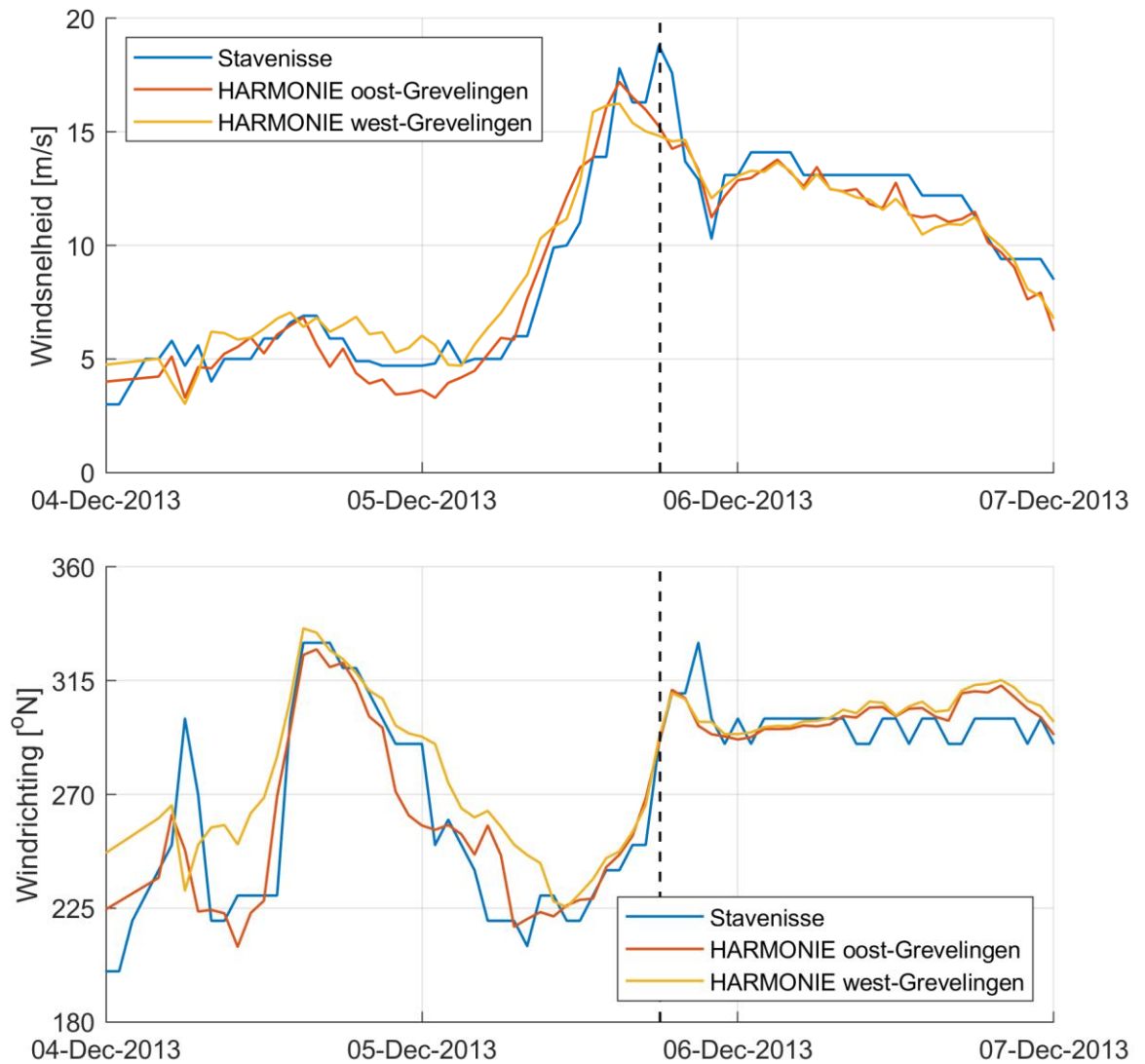
Figuur 5-7 Windsnelheid (m/s) en -richting (graden t.o.v. het Noorden) in meetstation Stavenisse en uit het KNMI HARMONIE-model tijdens de Sinterklaasstorm (december 2013)
