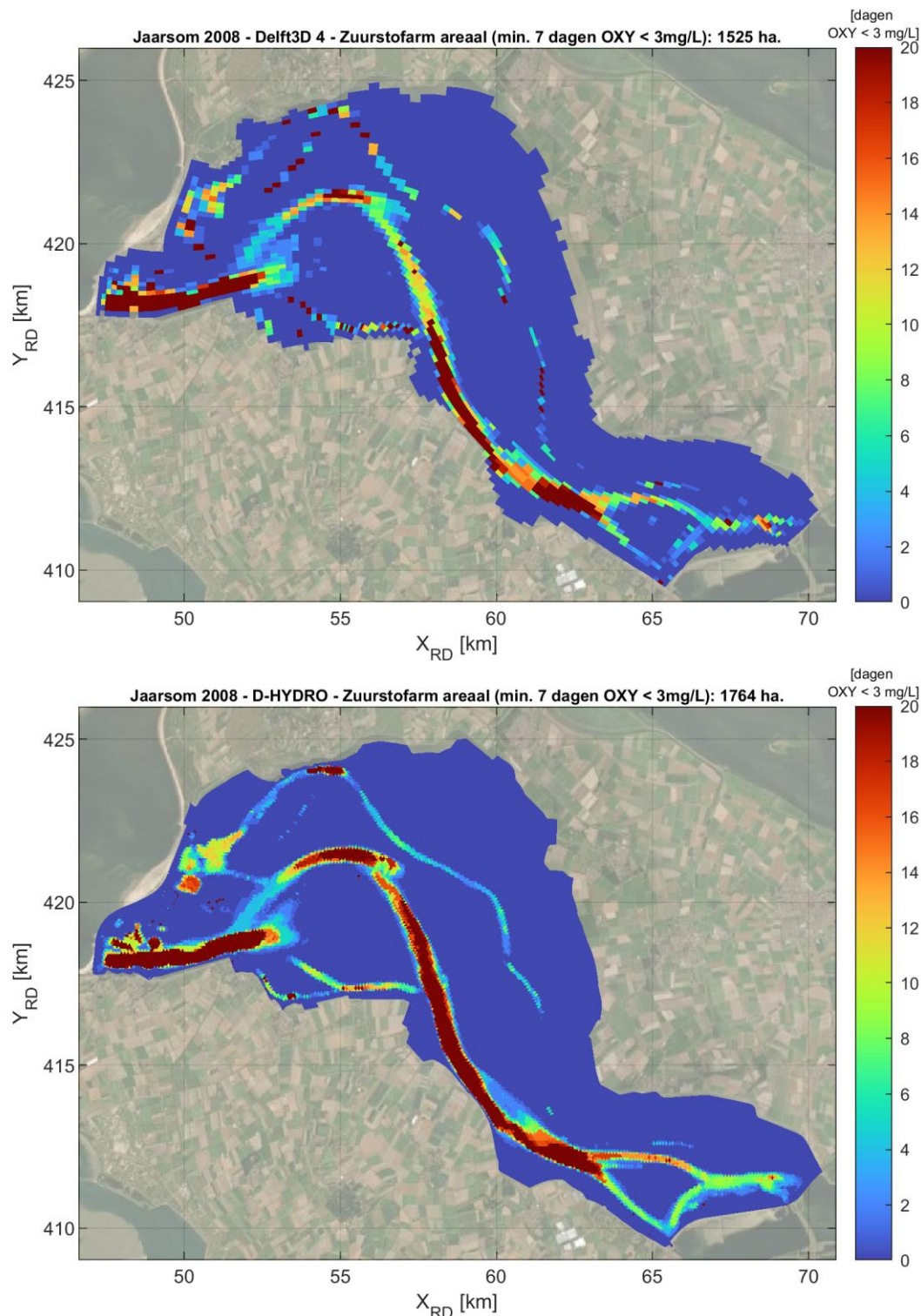
Figuur 8-18. Maximaal aantal aaneengesloten dagen van zuurstofarme condities (concentratie <math>< 3 \text{ mg/L}</math>) voor het Grevelingenmeer berekend met het Delft3D 4-model (bovenste paneel) en het D-HYDRO-model (onderste paneel). Het zuurstofarme areaal (in ha.) wordt berekend (zie waarde in titel) op basis van tenminste 7 aaneengesloten dagen van zuurstofarme condities.
