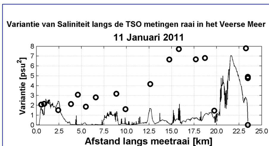
Figuur 5-12: Voorbeeld Variantie van Saliniteit (11 januari 2011) van metingen (bolletjes) en berekening. Oriëntatie is van West (Veerse Dam, 0 km) naar Oost (Zandkreekdijk, 22,5 km)
