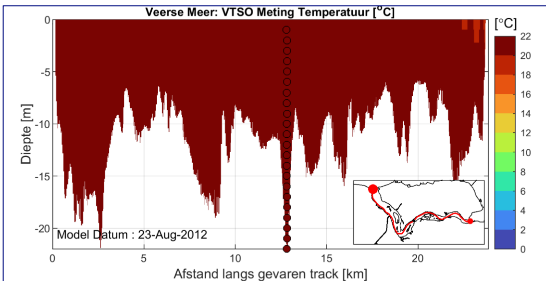
Figuur F-68: Temperatuur, TSO metingen Veers Meer; Meting tegen berekening 23 Augustus 2012
