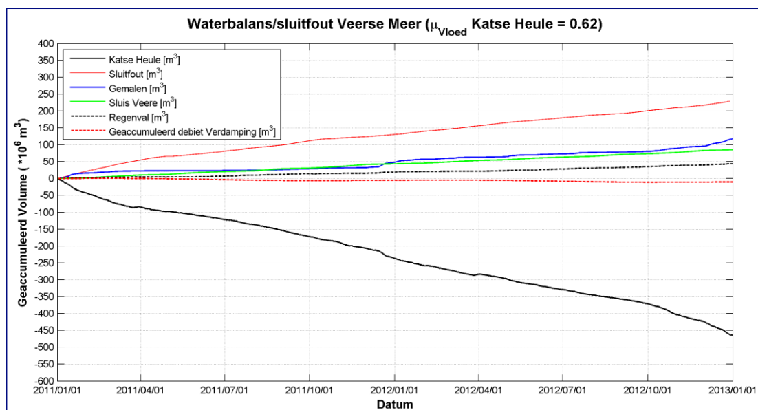
Figuur 5-2: Sluitfout waterbalans Veerse Meer in combinatie met afzonderlijke termen in de waterbalans ( \mu_{Vloed} = 0,62 )
