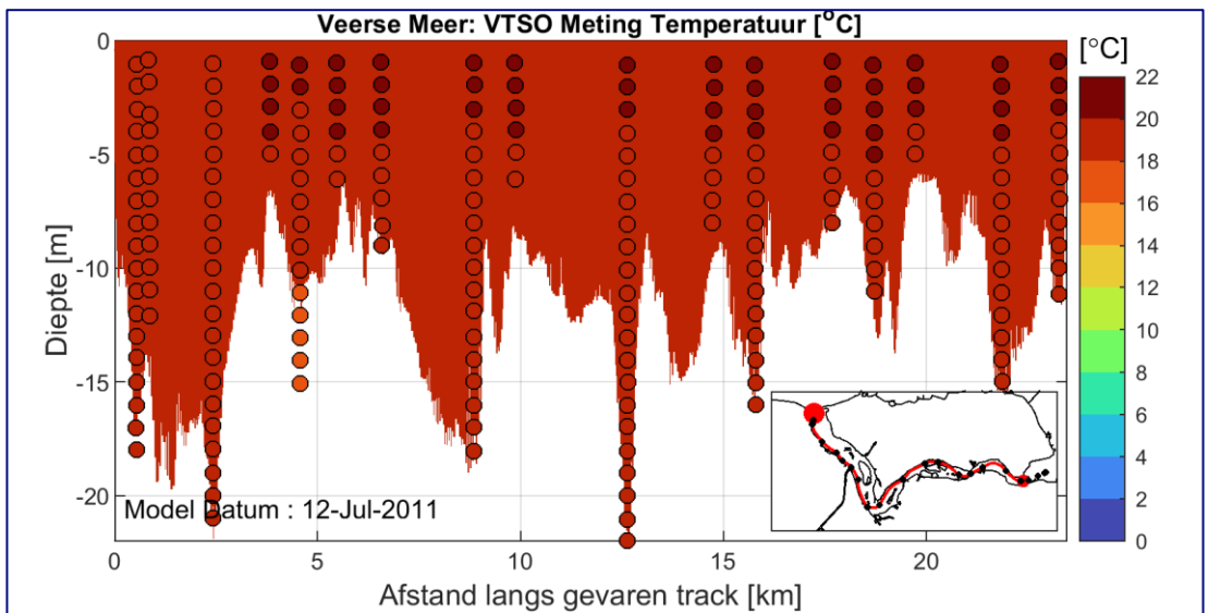
Figuur J-47: Temperatuur, TSO metingen Veers Meer; Meting tegen berekening 12 Juli 2011
