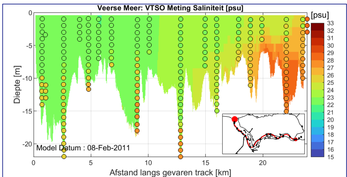
Figuur F-2: Saliniteit, TSO metingen Veerse Meer; Meting tegen berekening 8 Februari 2011
