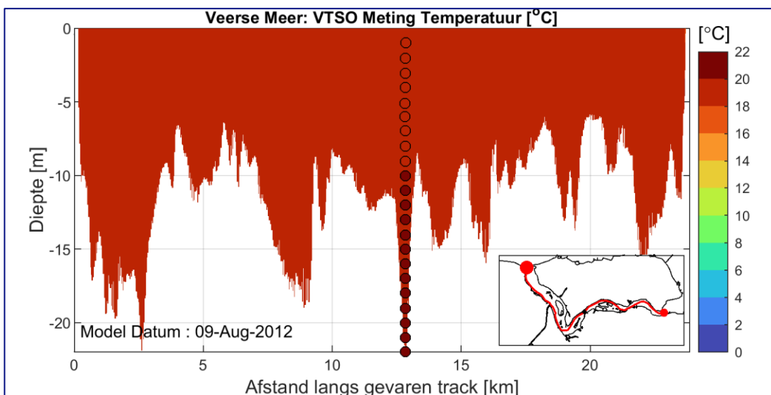
Figuur F-67: Temperatuur, TSO metingen Veers Meer; Meting tegen berekening 9 Augustus 2012
