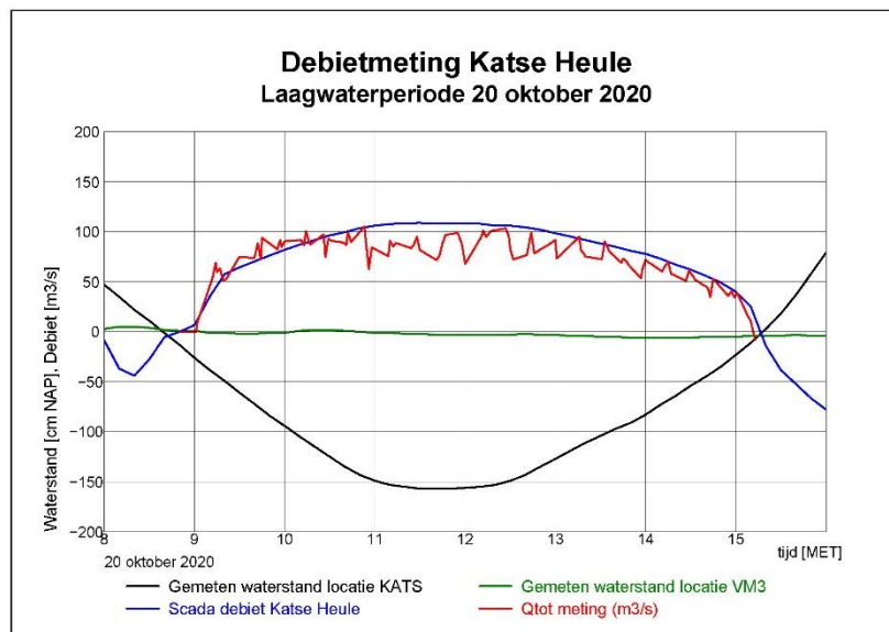
Figuur B3: Resultaten debietmeting spuien 20 oktober 2020.
