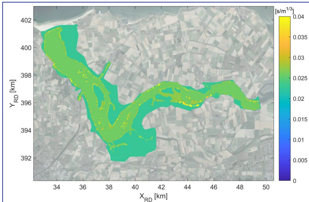
Figuur 4-3 Bodemruwheid (Manning-coëfficiënt)
