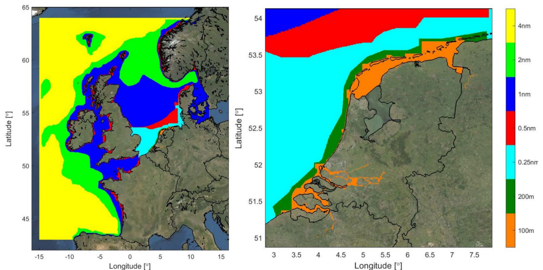
Figuur A-1 Domein van het DCSM-FM 100m model. Kleuren tonen de resolutie van het rooster (geel: ~4nm; licht groen: ~2nm; blauw: ~1nm; rood: 0.5 nm; cyaan: ~0.25 nm; donker groen: ~200m en oranje: ~100m).
