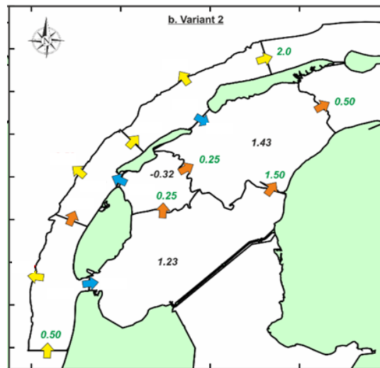
Figuur 2-24 Grootschalige sedimentbalans in de westelijke Waddenzee vanaf de jaren '90 volgens Elias (2019). De zwarte getallen geven de trends aan in miljoen m 3 /j en de groene getallen de transporten in miljoen m 3 /j.
