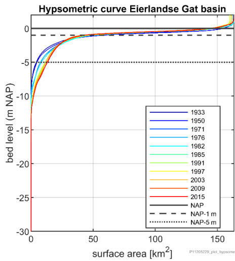
Figuur 2-28 Hypsometrische curven voor het bekken van het Eierlandse Gat voor verschillende jaren (links) en ingezoomd op deel tussen NAP-5 en NAP-1 m.
