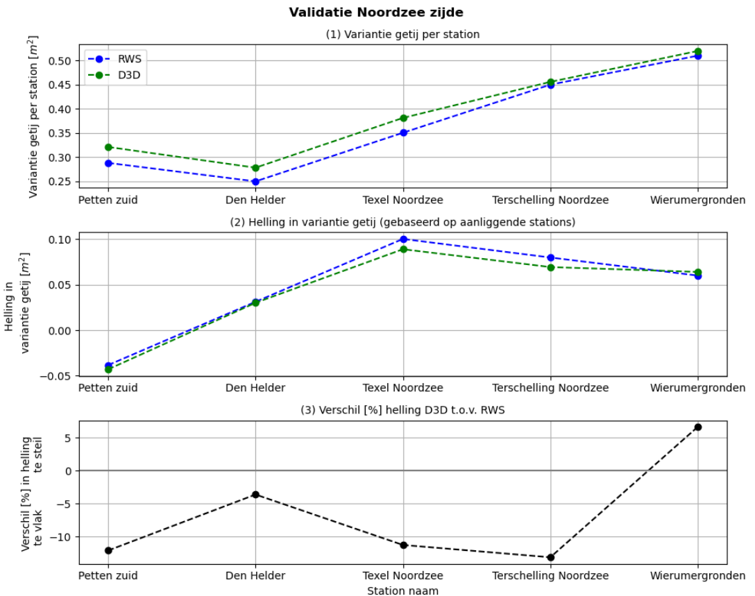
Figuur A-3 Vergelijking gemeten en berekende (gradiënten in) getijamplitude langs de zeegaten. Blauwe stippen zijn Rijkswaterstaat metingen uit het jaar 2017, groene stippen tonen modeluitvoer voor de simulatie met randvoorwaarden uit 2017 en een bodem uit 2015. (1) Bovenste grafiek toont de variantie [m 2 ] van het
