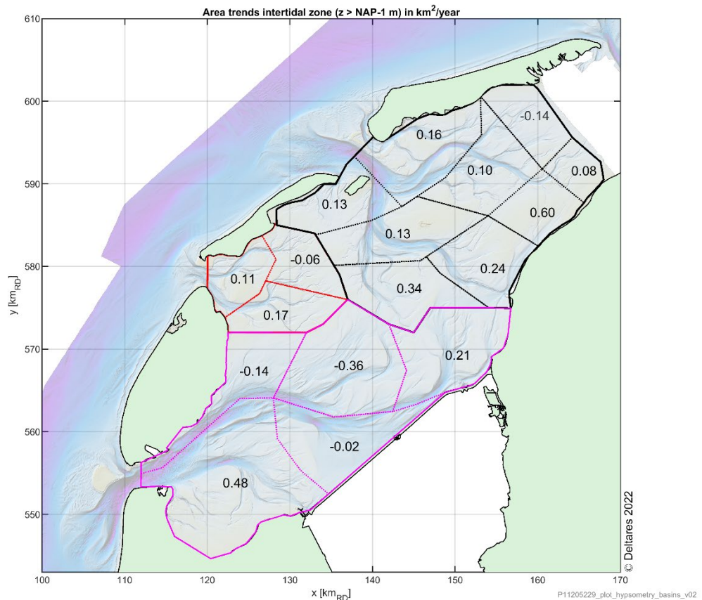
Figuur 2-31 Oppervlaktetrends in km 2 /jaar van de platen (z > NAP-1 m) in deelgebieden
