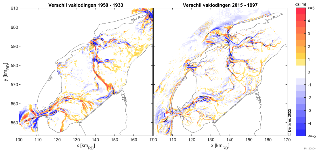
Figuur 2-18 Verschilkaart vaklodgingen 1950 - 1933 (17 jaar) en 2015 - 1997 (18 jaar).
