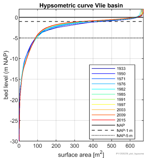
Figuur 2-29 Hypsometrische curven voor het bekken van het Zeegat van het Vlie voor verschillende jaren (links) en ingezoomd op deel tussen NAP-5 en NAP-1 m.
