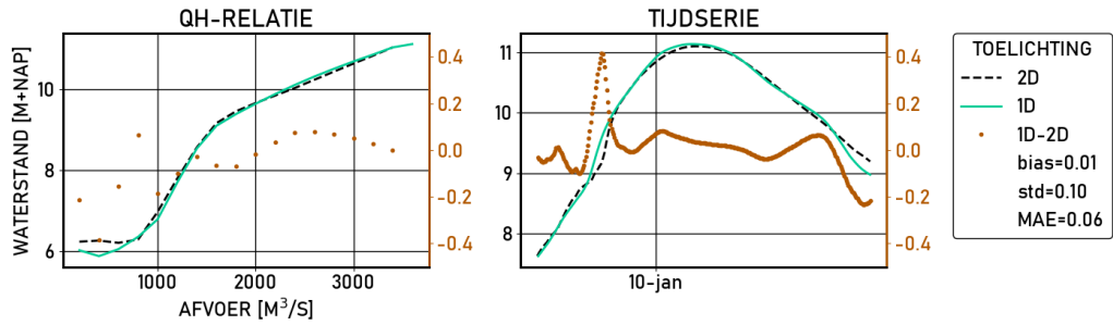
Figure 2.437 Grebbe | figures | Validatie | D16000 | stations
