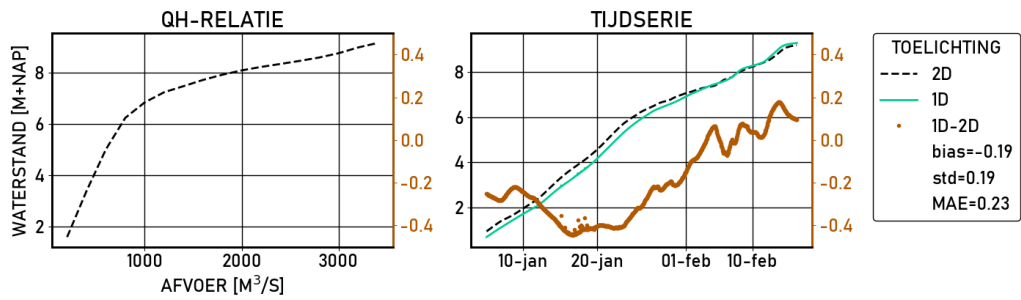
Figure 2.177 Eefde-beneden | figures | Ongekalibreerd | stations
