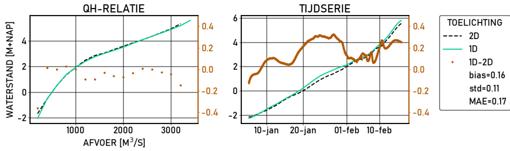
Figure 2.241 Katerveer | figures | Ongekalibreerd | stations
