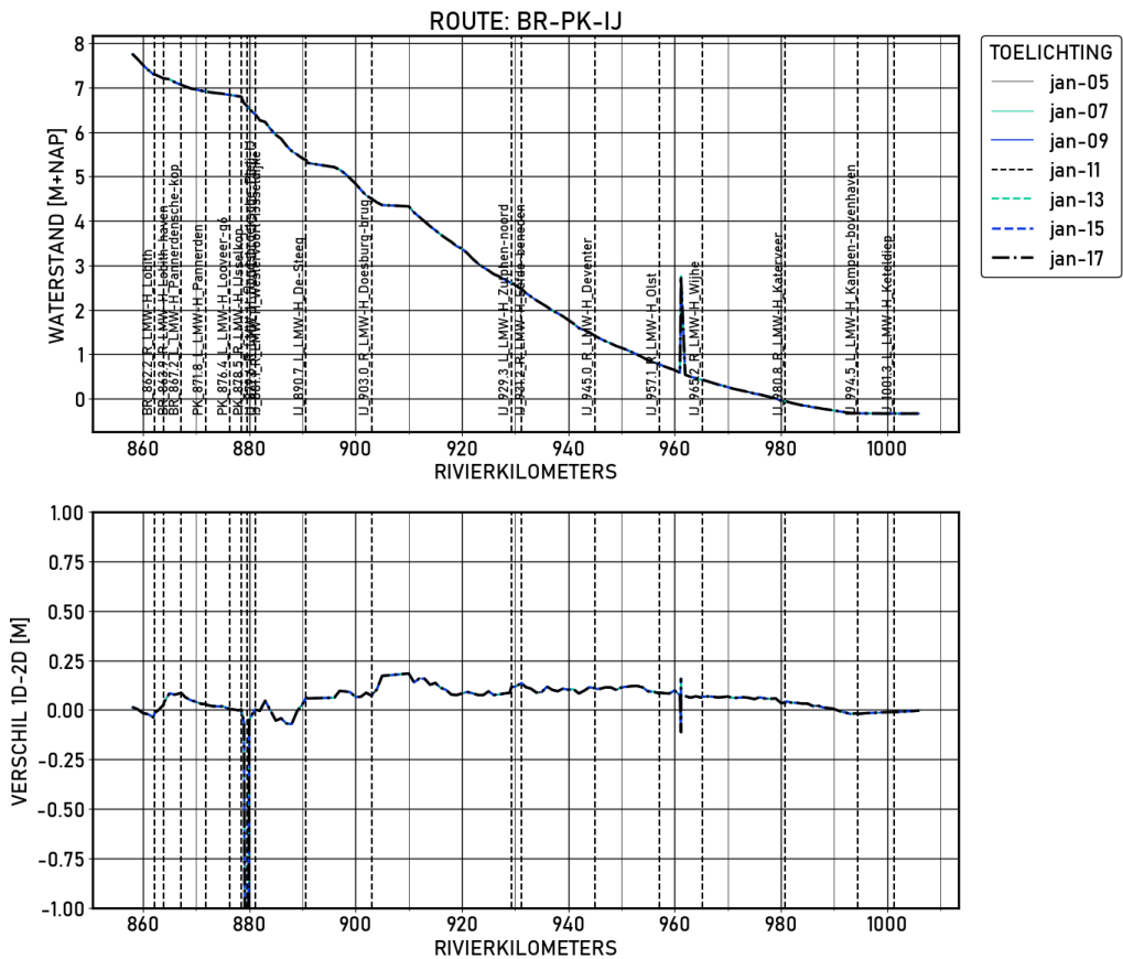
Figure 1.21 BR-PK-IJ | figures | Validatie | S_1020 | Langsprofiel
