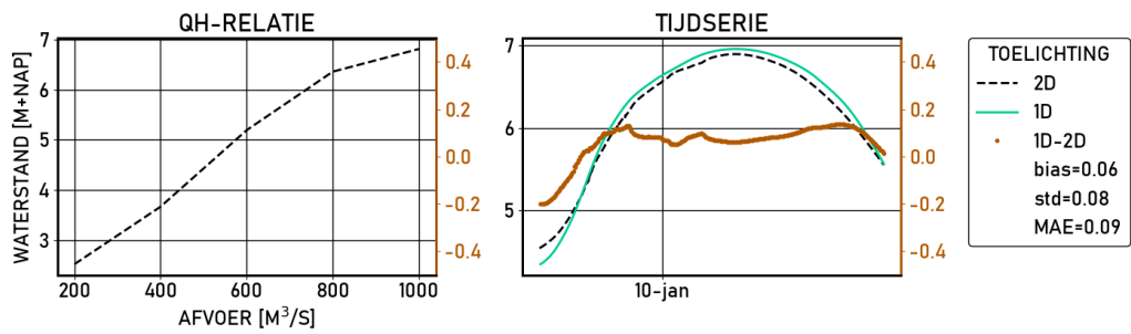
Figure 2.182 Eefde-beneden | figures | Validatie | D_6000 | stations
