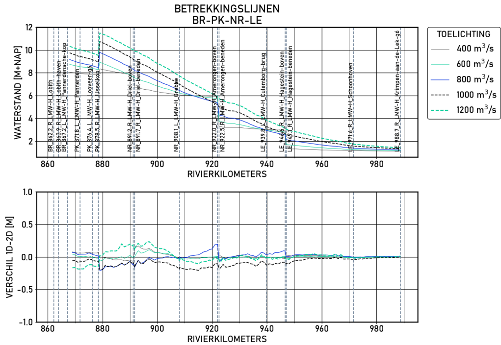
Figure 1.76 BR-PK-NR-LE | figures | Validatie | D_6000 | Langsprofiel
