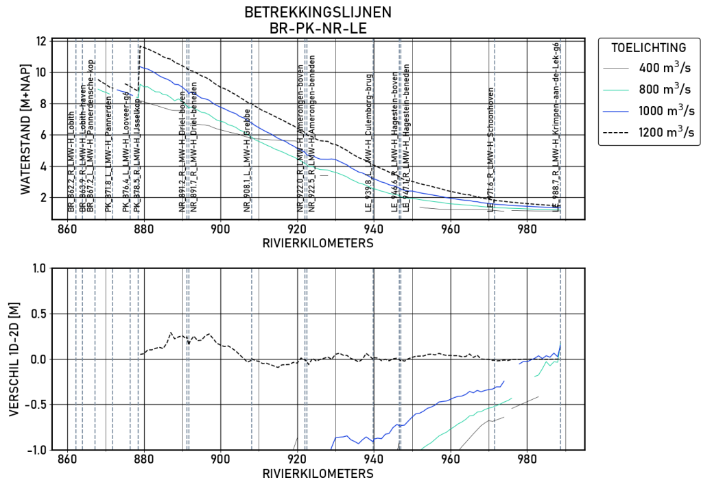
Figure 1.92 BR-PK-NR-LE | figures | Validatie | S_6000 | Langsprofiel
