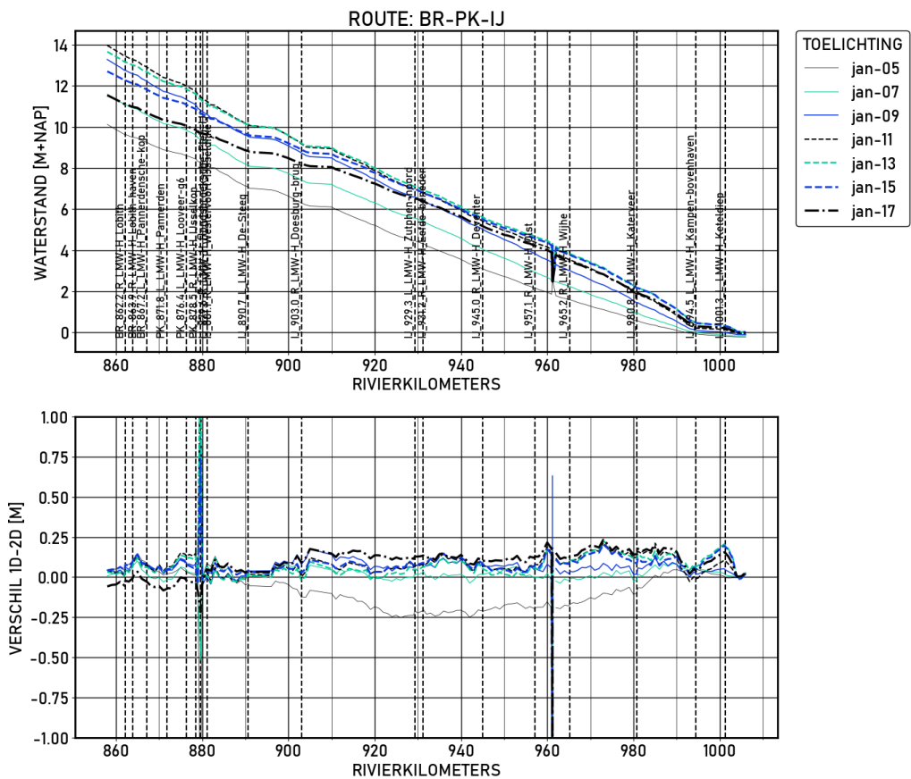
Figure 1.11 BR-PK-IJ | figures | Validatie | D_6000 | Langsprofiel
