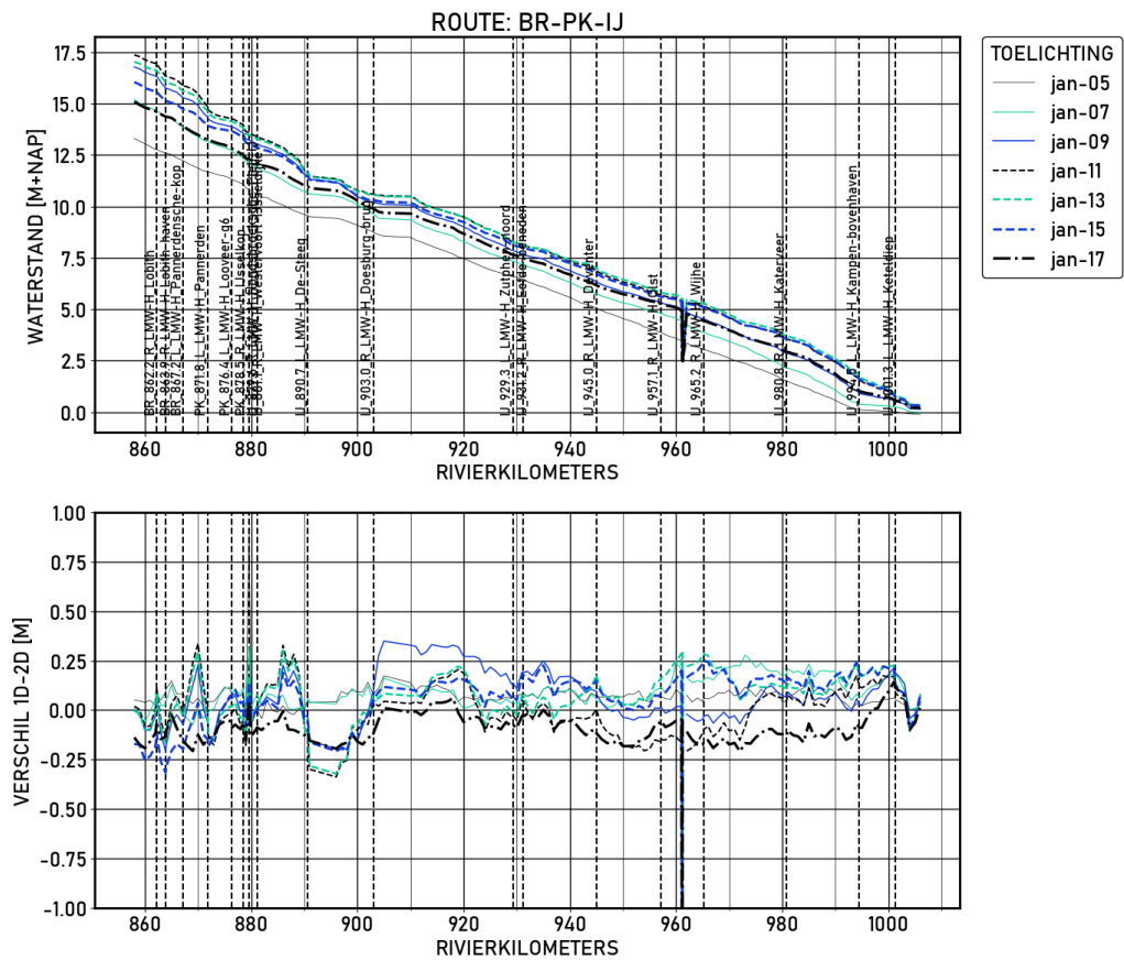
Figure 1.7 BR-PK-IJ | figures | Validatie | D13000 | Langsprofiel
