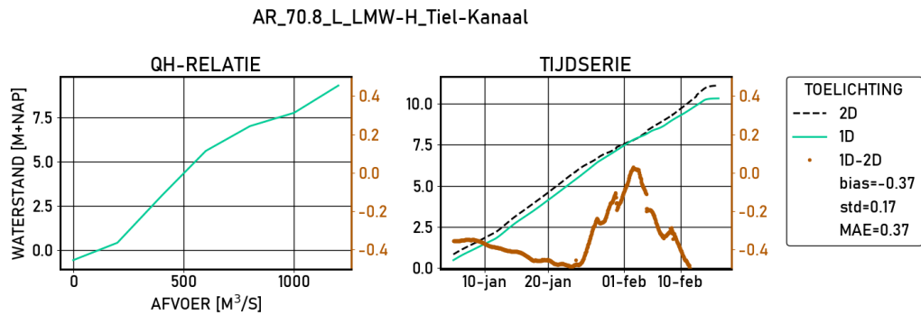
Figure 2.1 Tiel-Kanaal | figures | Ongekalibreerd | stations
