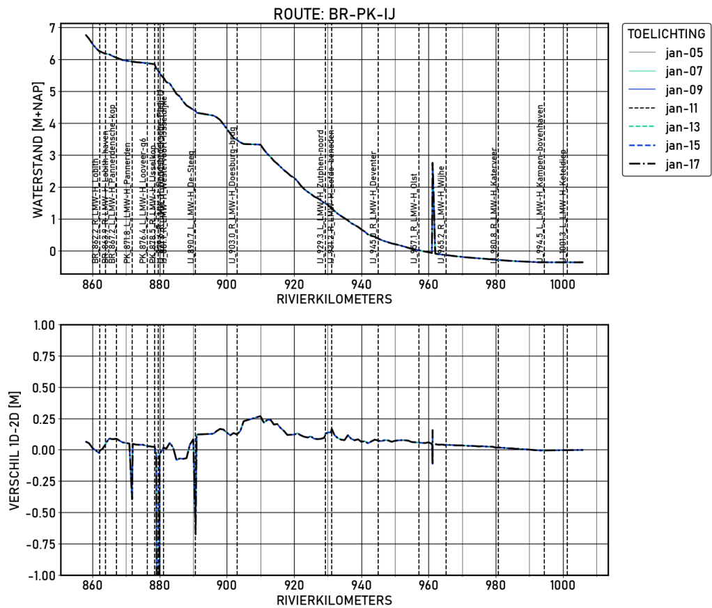
Figure 1.31 BR-PK-IJ | figures | Validatie | S_600 | Langsprofiel
