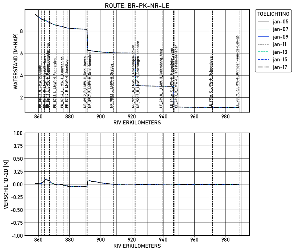
Figure 1.87 BR-PK-NR-LE | figures | Validatie | S_2000 | Langsprofiel
