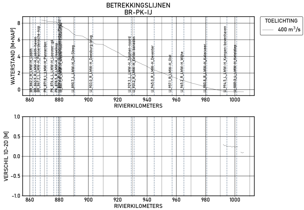
Figure 1.32 BR-PK-IJ | figures | Validatie | S_600 | Langsprofiel
