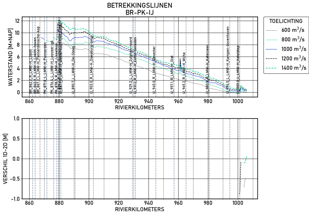
Figure 1.20 BR-PK-IJ | figures | Validatie | S16000 | Langsprofiel
