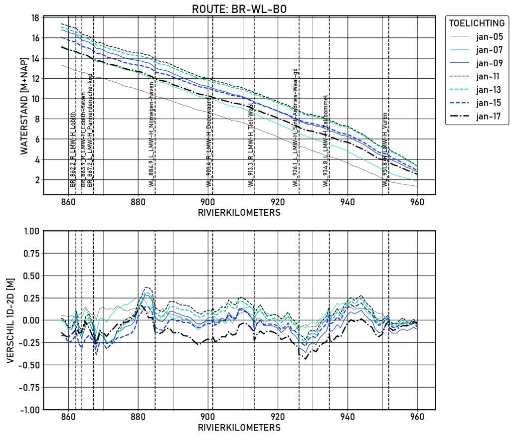
Figure 1.39 BR-WL-B0 | figures | Validatie | D13000 | Langsprofiel
