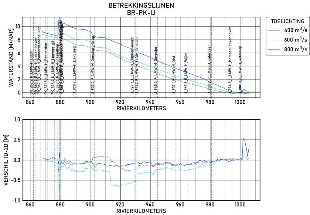
Figure 1.6 BR-PK-IJ | figures | Validatie | D10000 | Langsprofiel
