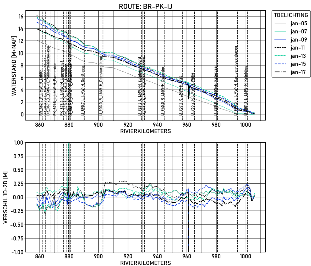
Figure 1.5 BR-PK-IJ | figures | Validatie | D10000 | Langsprofiel
