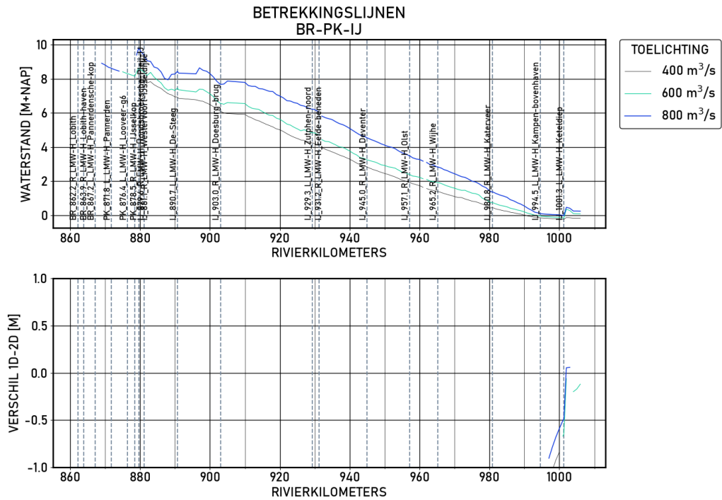
Figure 1.16 BR-PK-IJ | figures | Validatie | S10000 | Langsprofiel
