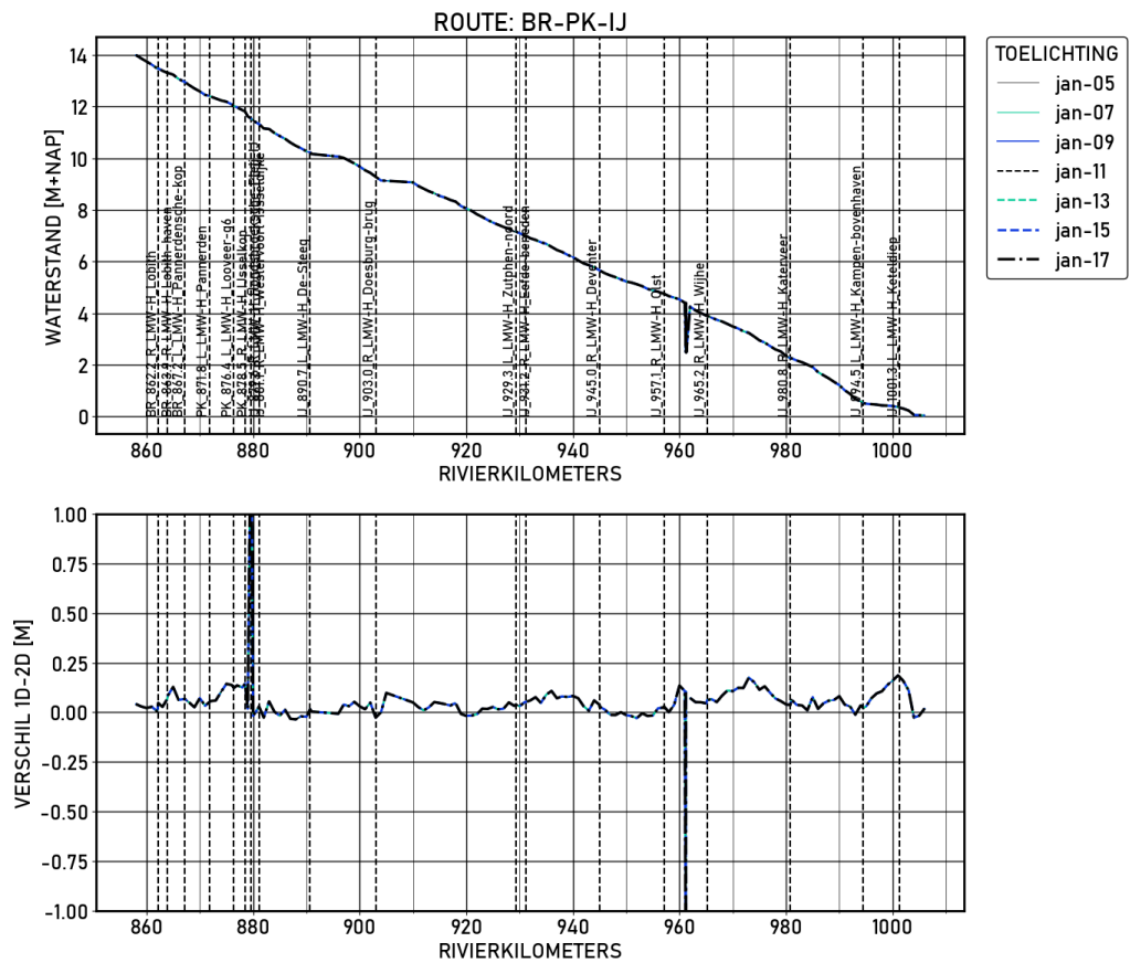
Figure 1.27 BR-PK-IJ | figures | Validatie | S_600 | Langsprofiel
