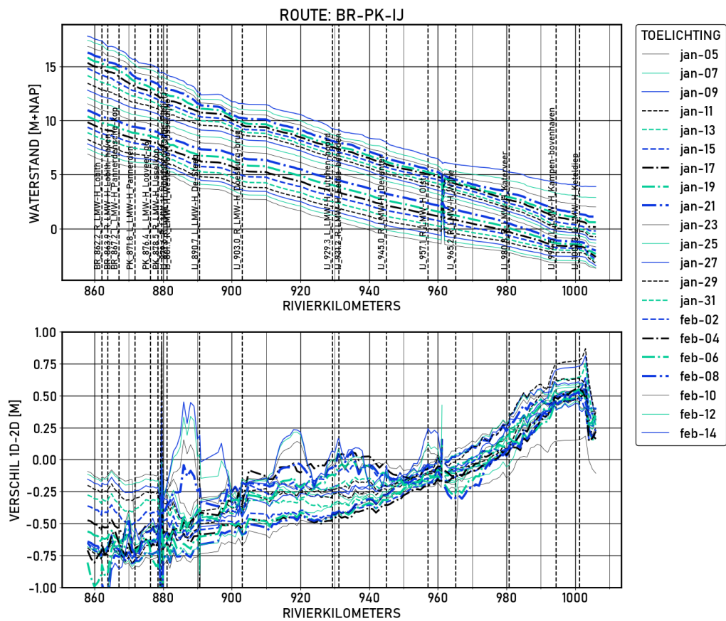
Figure 1.1 BR-PK-IJ | figures | Ongekalibreerd | Langsprofiel
