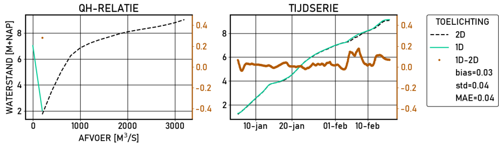
Figure 2.178 Eefde-beneden | figures | Kalibratie | stations
