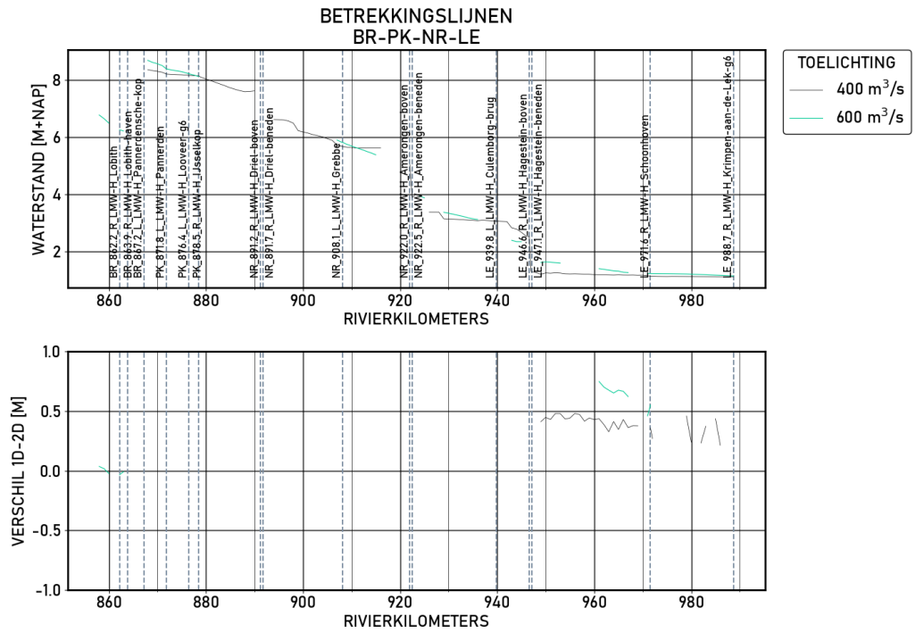
Figure 1.96 BR-PK-NR-LE | figures | Validatie | S_600 | Langsprofiel
