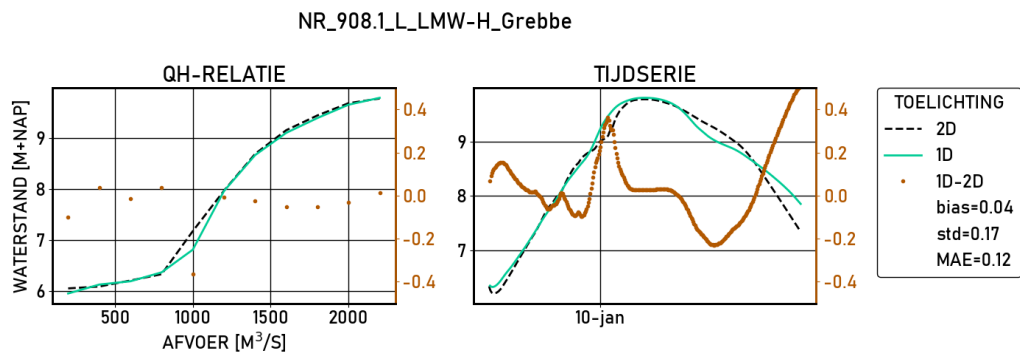
Figure 2.435 Grebbe | figures | Validatie | D10000 | stations
