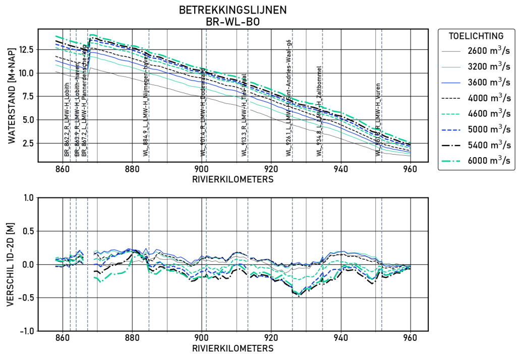
Figure 1.38 BR-WL-B0 | figures | Validatie | D10000 | Langsprofiel
