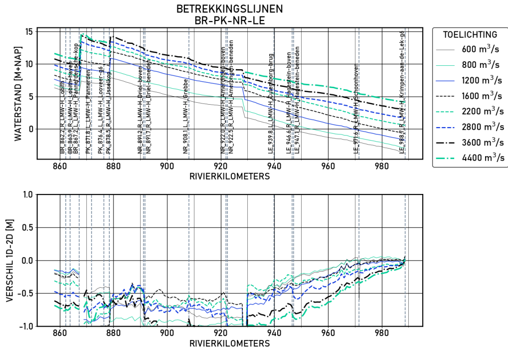
Figure 1.66 BR-PK-NR-LE | figures | Ongekalibreerd | Langsprofiel
