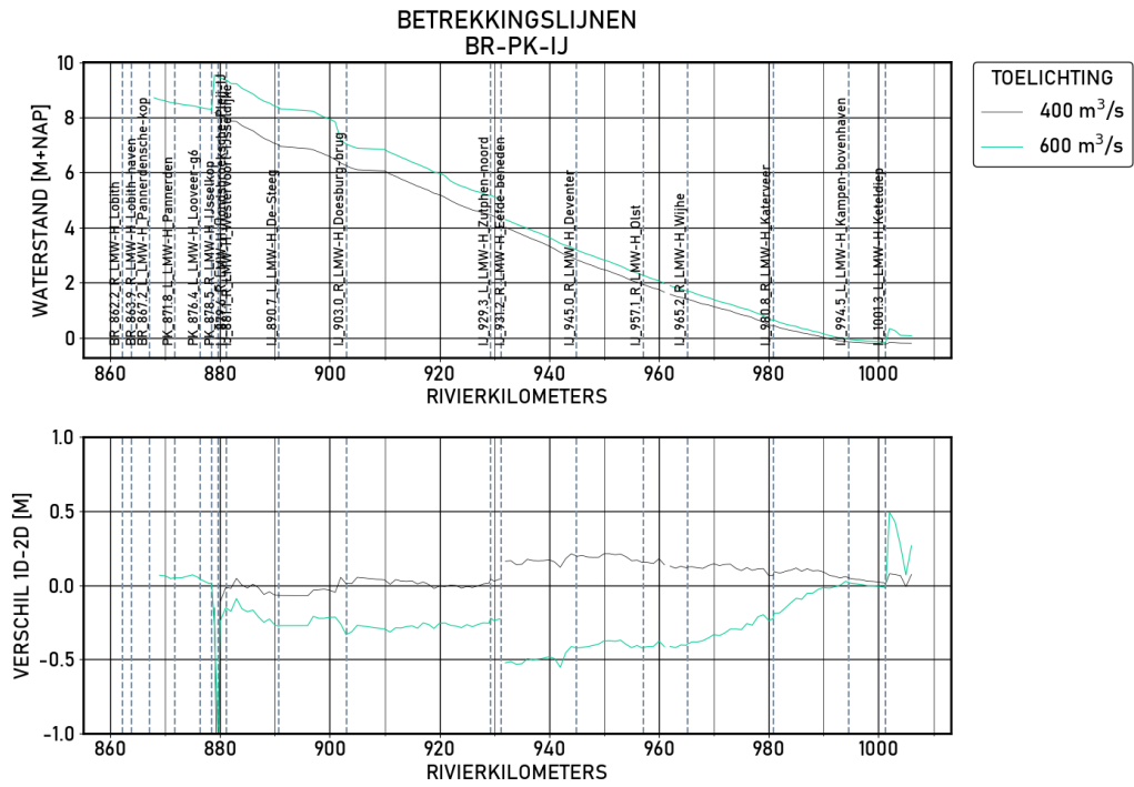
Figure 1.14 BR-PK-IJ | figures | Validatie | D_8000 | Langsprofiel
