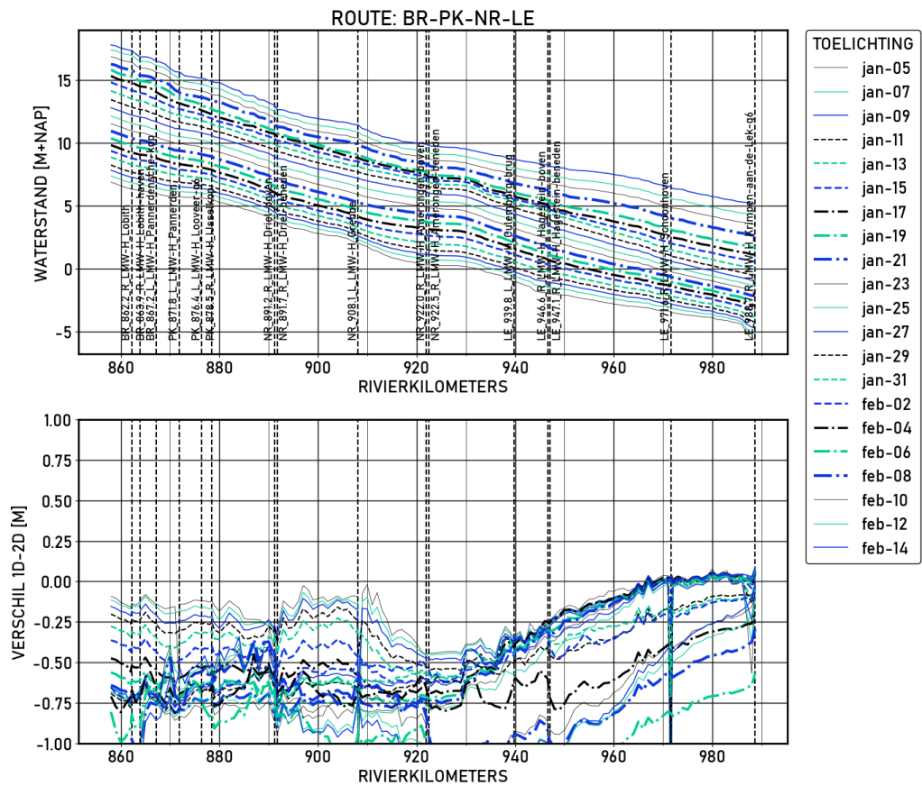
Figure 1.65 BR-PK-NR-LE | figures | Ongekalibreerd | Langsprofiel
