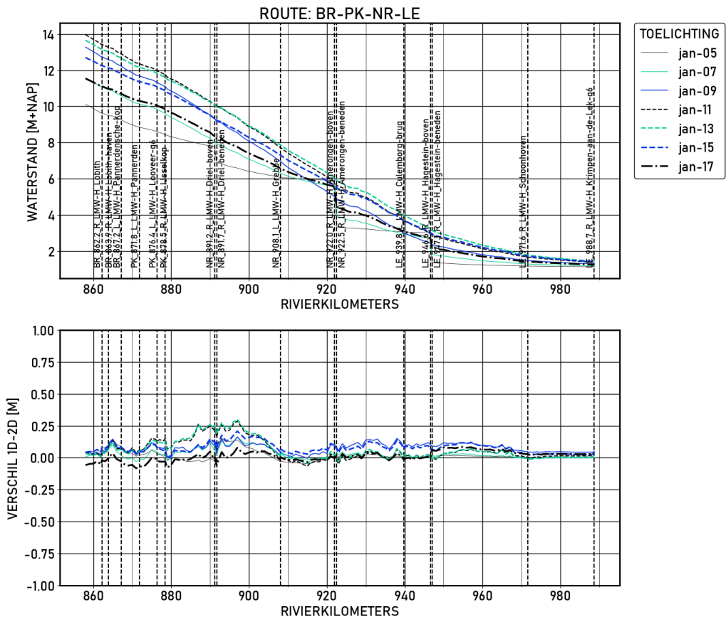
Figure 1.75 BR-PK-NR-LE | figures | Validatie | D_6000 | Langsprofiel
