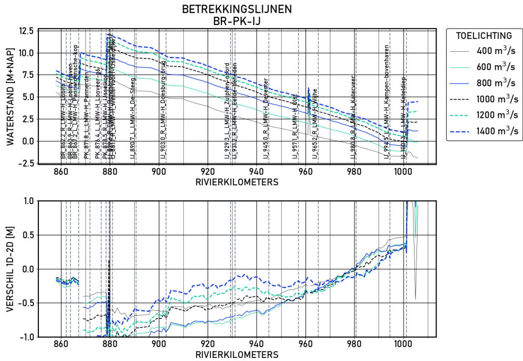
Figure 1.2 BR-PK-IJ | figures | Ongekalibreerd | Langsprofiel
