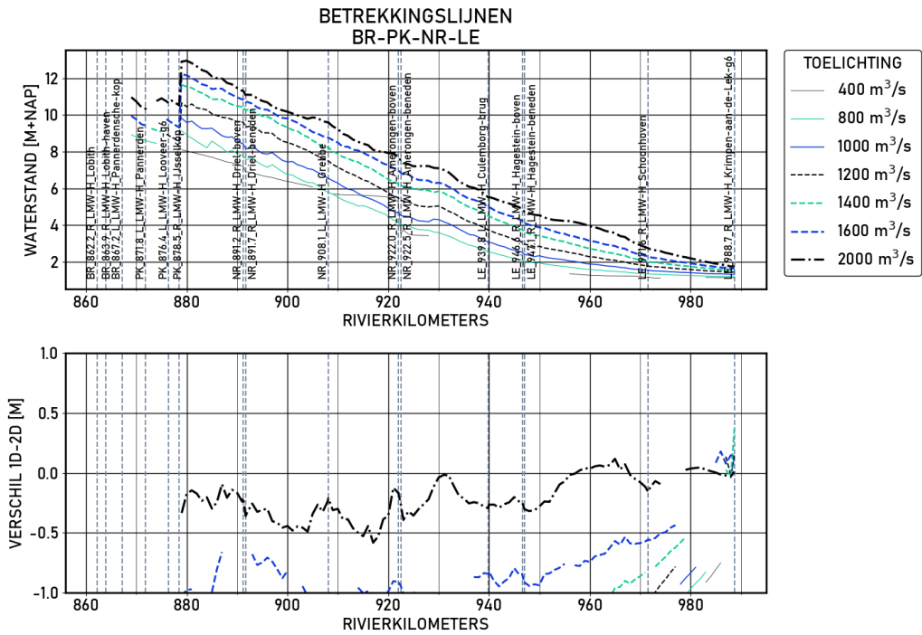
Figure 1.80 BR-PK-NR-LE | figures | Validatie | S10000 | Langsprofiel
