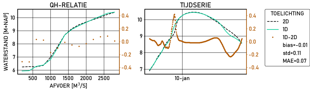
Figure 2.436 Grebbe | figures | Validatie | D13000 | stations
