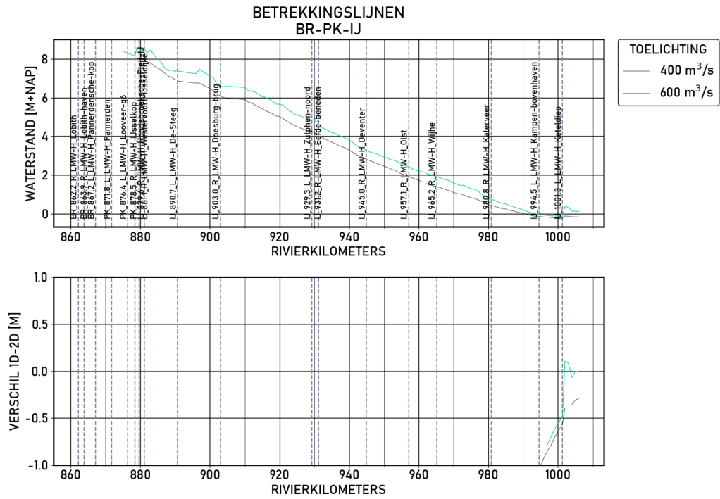
Figure 1.30 BR-PK-IJ | figures | Validatie | S_8000 | Langsprofiel
