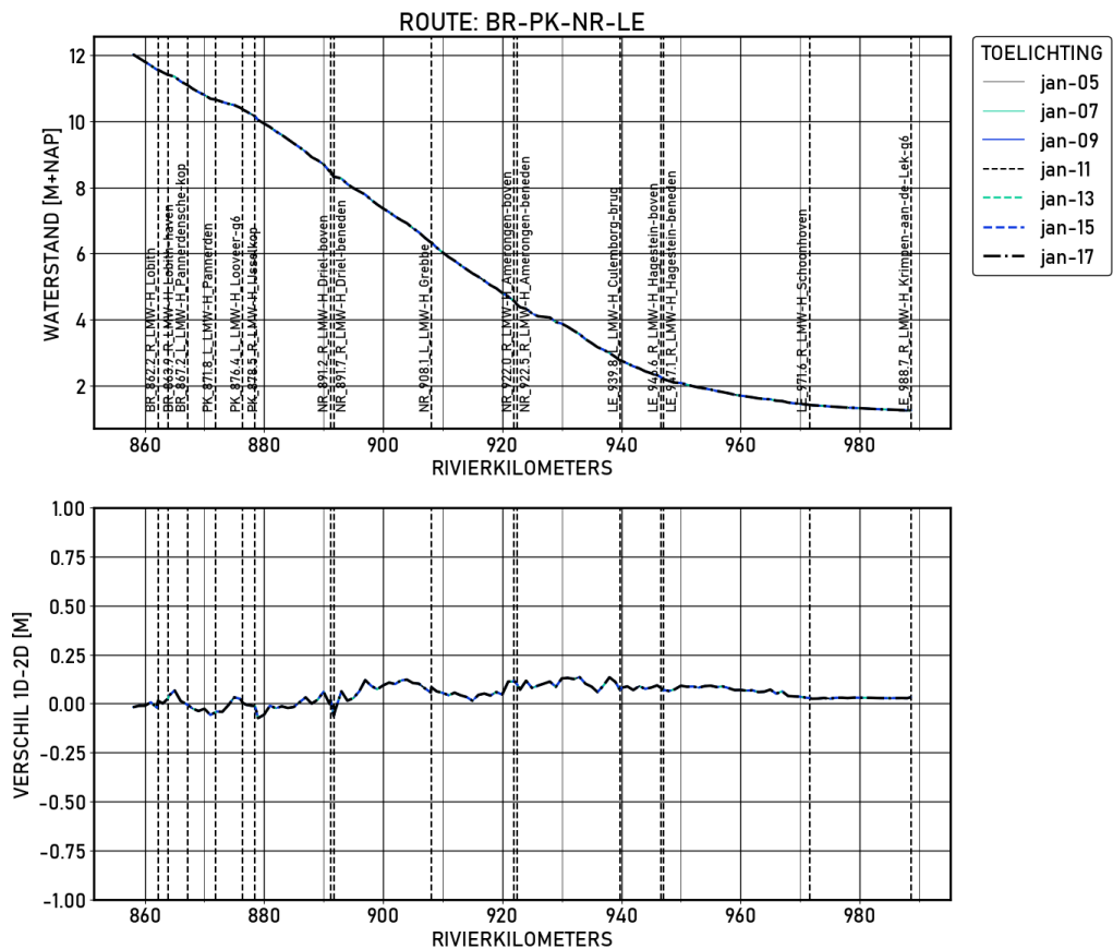
Figure 1.89 BR-PK-NR-LE | figures | Validatie | S_4000 | Langsprofiel
