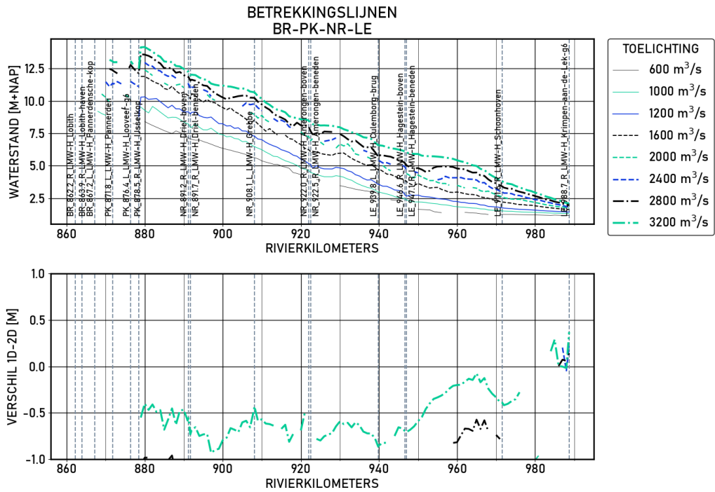
Figure 1.84 BR-PK-NR-LE | figures | Validatie | S16000 | Langsprofiel
