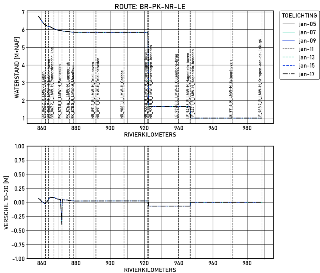
Figure 1.95 BR-PK-NR-LE | figures | Validatie | S_600 | Langsprofiel
