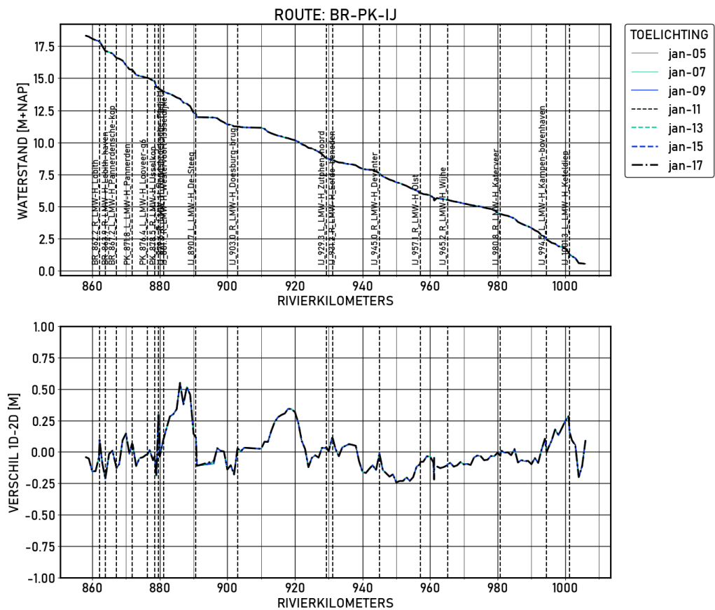
Figure 1.19 BR-PK-IJ | figures | Validatie | S16000 | Langsprofiel
