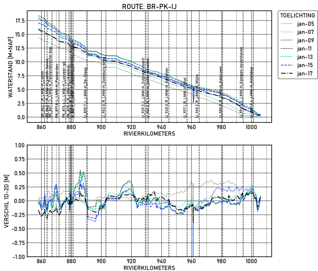
Figure 1.9 BR-PK-IJ | figures | Validatie | D16000 | Langsprofiel
