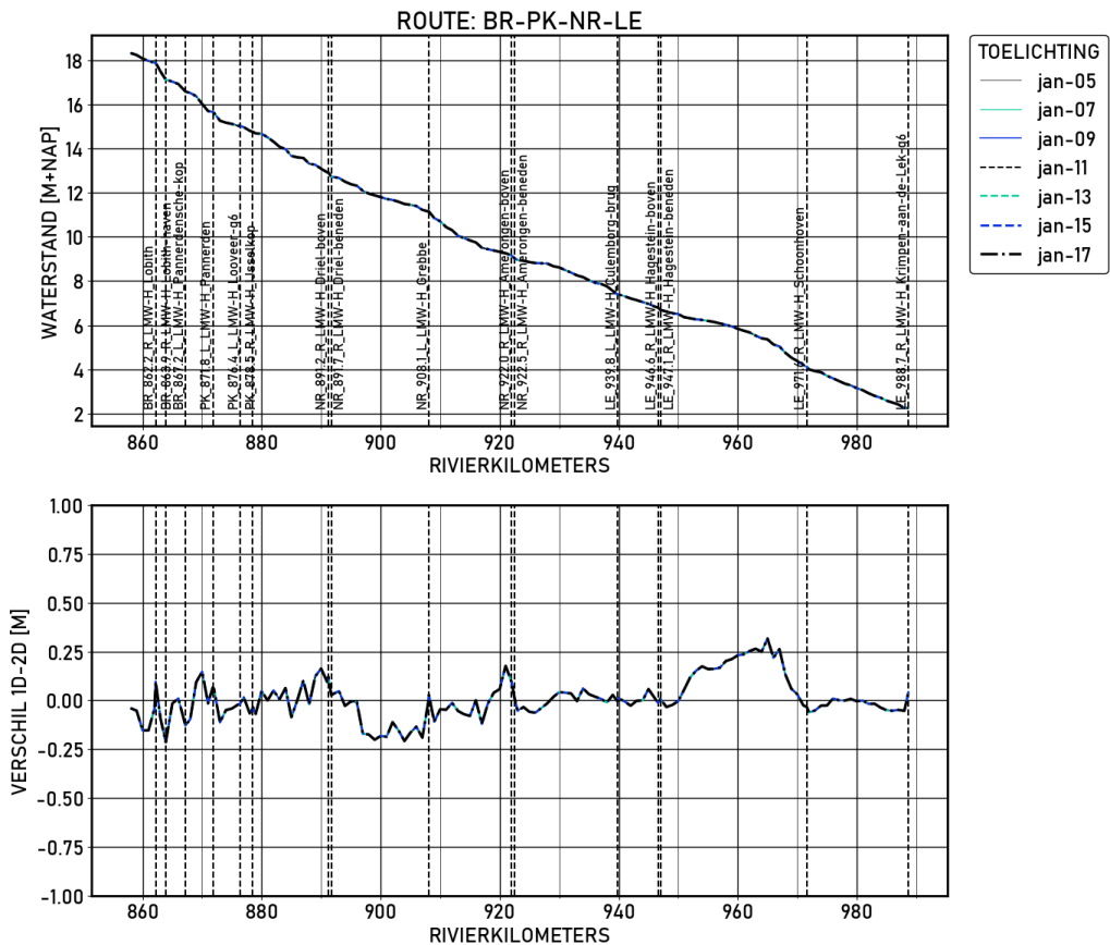
Figure 1.83 BR-PK-NR-LE | figures | Validatie | S16000 | Langsprofiel
