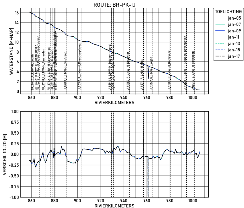
Figure 1.15 BR-PK-IJ | figures | Validatie | S10000 | Langsprofiel
