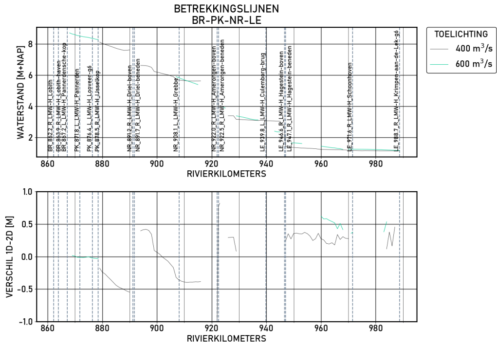
Figure 1.88 BR-PK-NR-LE | figures | Validatie | S_2000 | Langsprofiel
