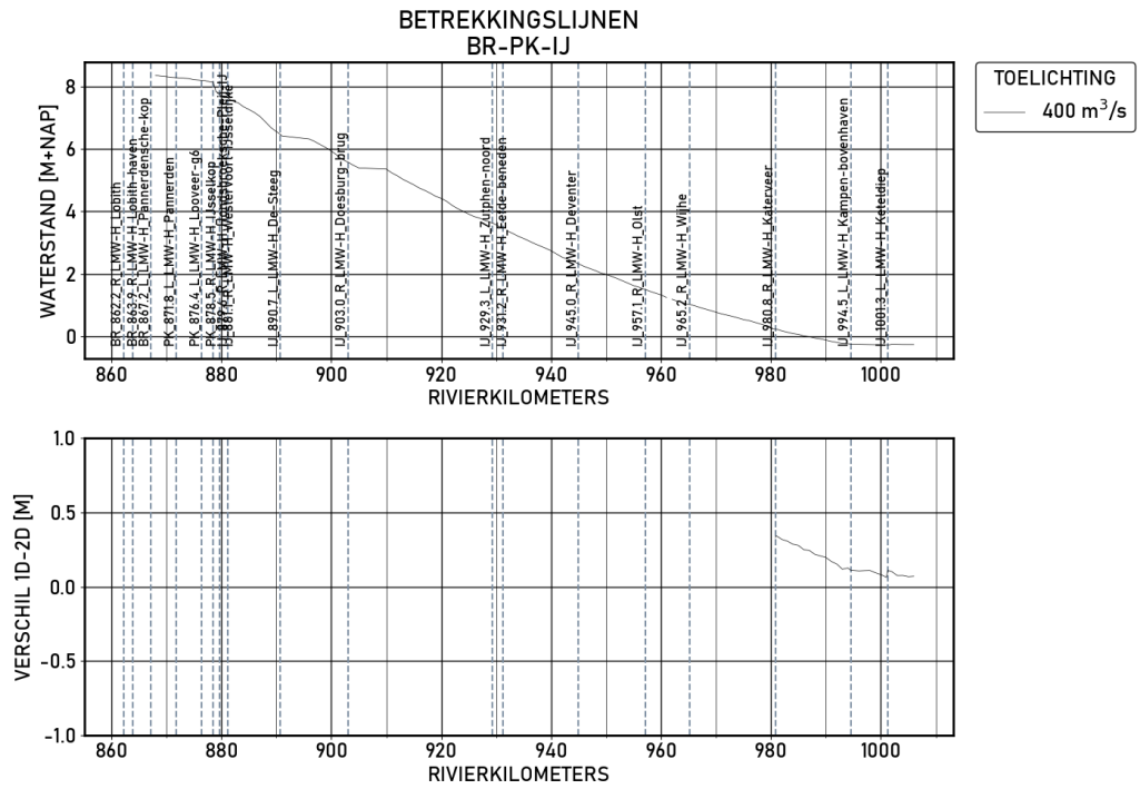
Figure 1.22 BR-PK-IJ | figures | Validatie | S_1020 | Langsprofiel
