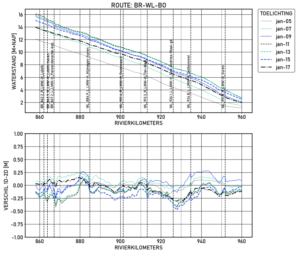
Figure 1.37 BR-WL-B0 | figures | Validatie | D10000 | Langsprofiel
