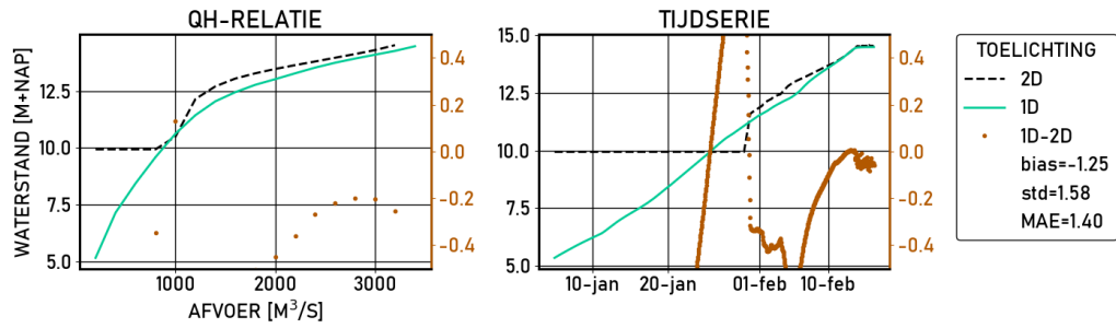
Figure 2.97 Hondsbroeksche-Pleij-IJ | figures | Ongekalibreerd | stations
