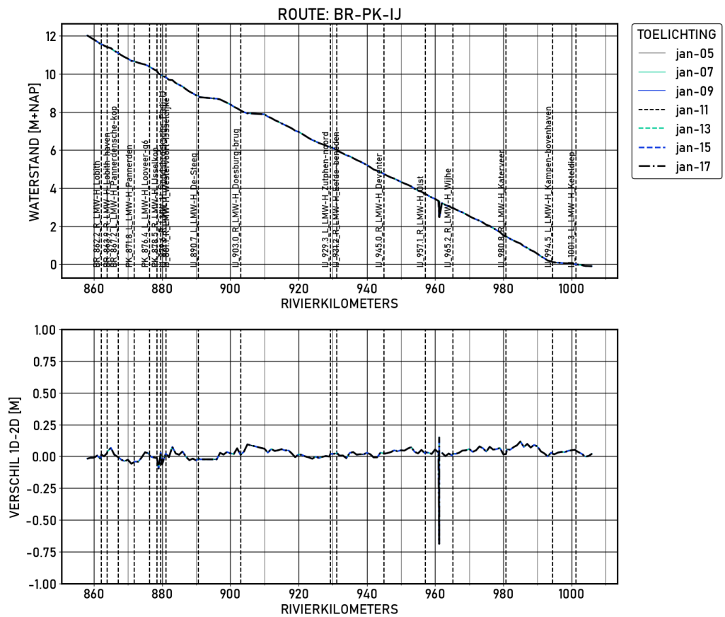
Figure 1.25 BR-PK-IJ | figures | Validatie | S_4000 | Langsprofiel
