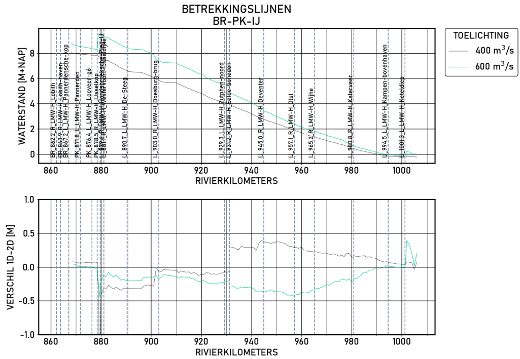
Figure 1.12 BR-PK-IJ | figures | Validatie | D_6000 | Langsprofiel
