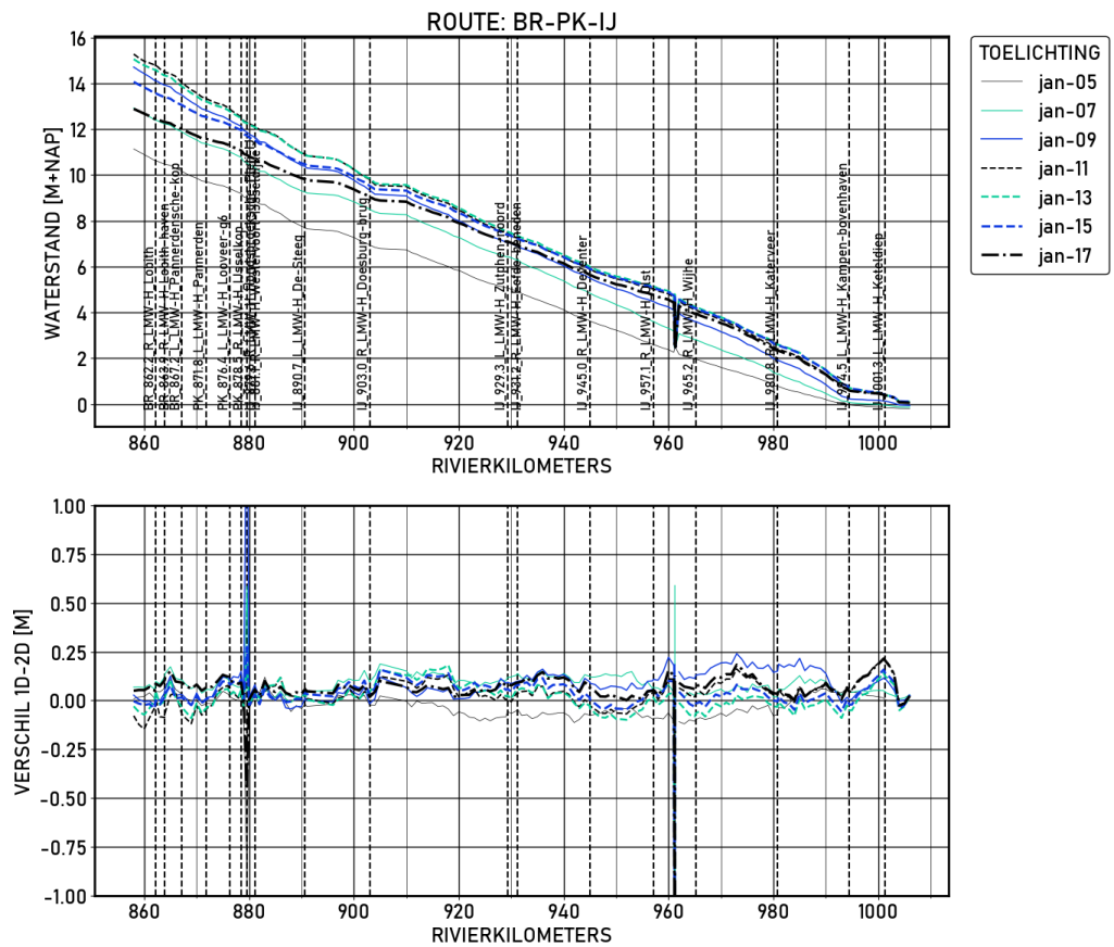
Figure 1.13 BR-PK-IJ | figures | Validatie | D_8000 | Langsprofiel
