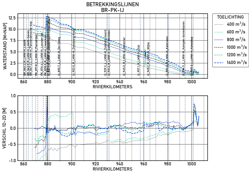
Figure 1.10 BR-PK-IJ | figures | Validatie | D16000 | Langsprofiel
