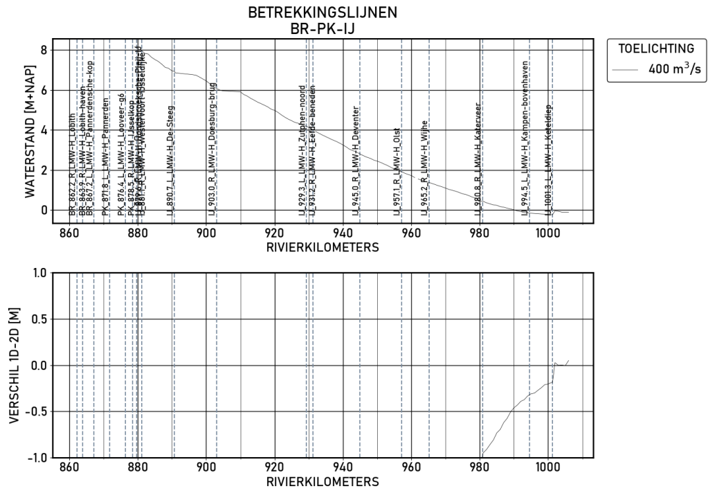
Figure 1.26 BR-PK-IJ | figures | Validatie | S_400 | Langsprofiel
