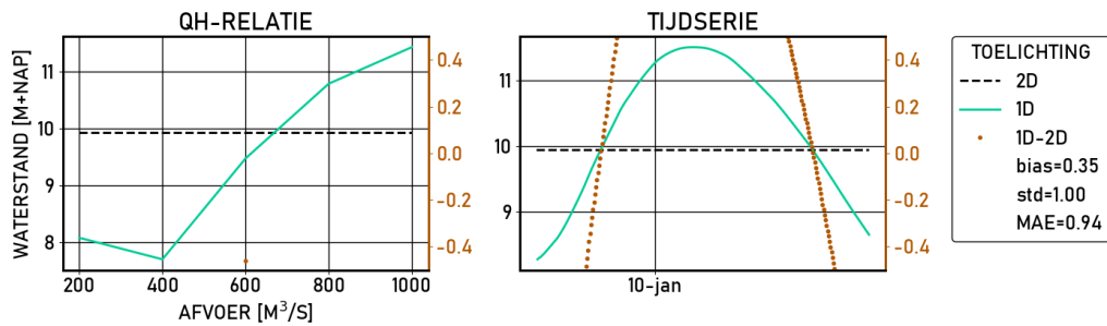
Figure 2.102 Hondsbroeksche-Pleij-IJ | figures | Validatie | D_6000 | stations
