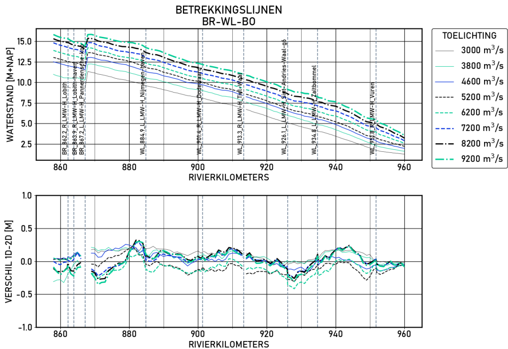
Figure 1.42 BR-WL-B0 | figures | Validatie | D16000 | Langsprofiel
