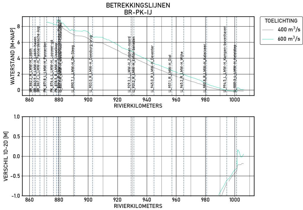
Figure 1.28 BR-PK-IJ | figures | Validatie | S_6000 | Langsprofiel
