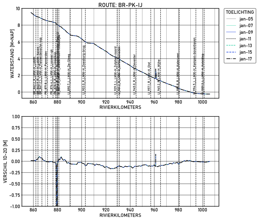
Figure 1.23 BR-PK-IJ | figures | Validatie | S_2000 | Langsprofiel
