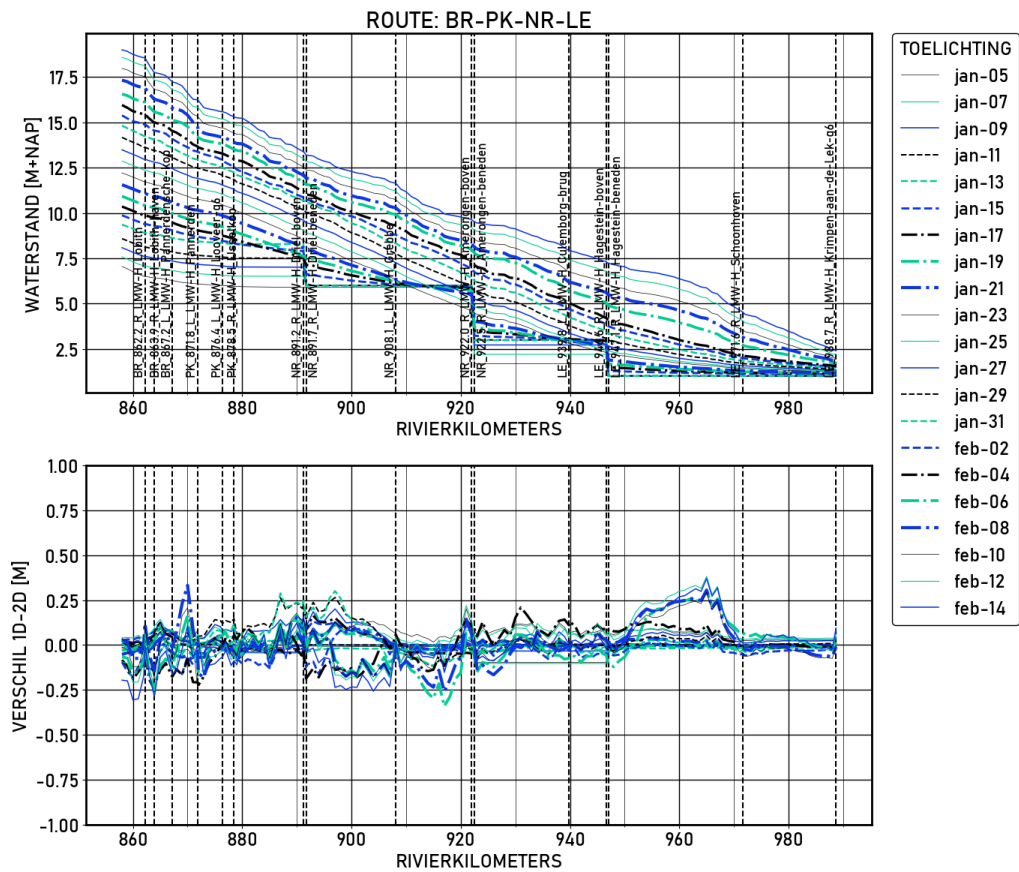
Figure 1.67 BR-PK-NR-LE | figures | Kalibratie | Langsprofiel
