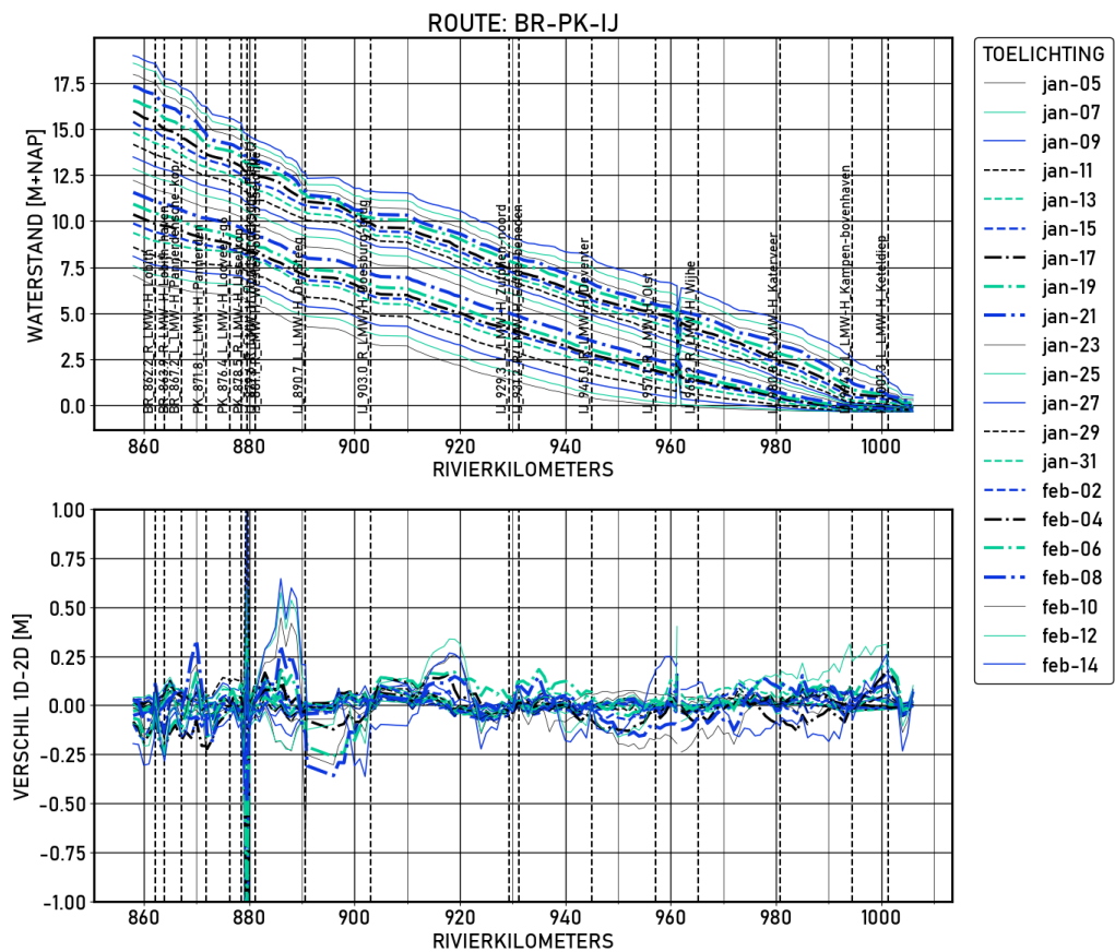
Figure 1.3 BR-PK-IJ | figures | Kalibratie | Langsprofiel
