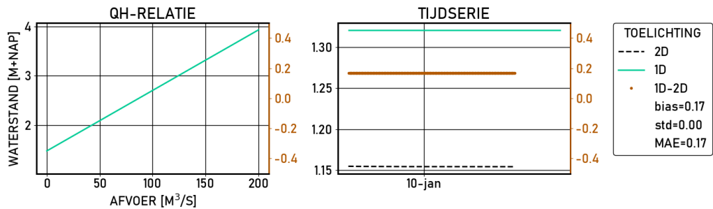
Figure 2.192 Eefde-beneden | figures | Validatie | S__600 | stations
