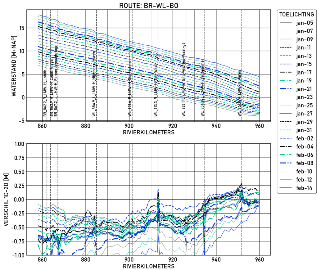
Figure 1.33 BR-WL-B0 | figures | Ongekalibreerd | Langsprofiel
