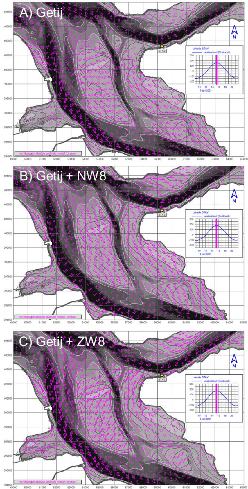
Figuur 3-8. Stromingssimulaties op de Galgeplaat met het SIMONA-Scaaloost model voor 9 juni 2021 15h20 op de 2019-bodem (Rijkswaterstaat, Kerst Buis). De kenmerkende stroming (richting + grootte) bij maximaal hoogwater is weergegeven voor een situatie met a) alleen getij, b) getij + noordwestenwind met windkracht 8 en c) getij + zuidwestenwind met windkracht 8.
