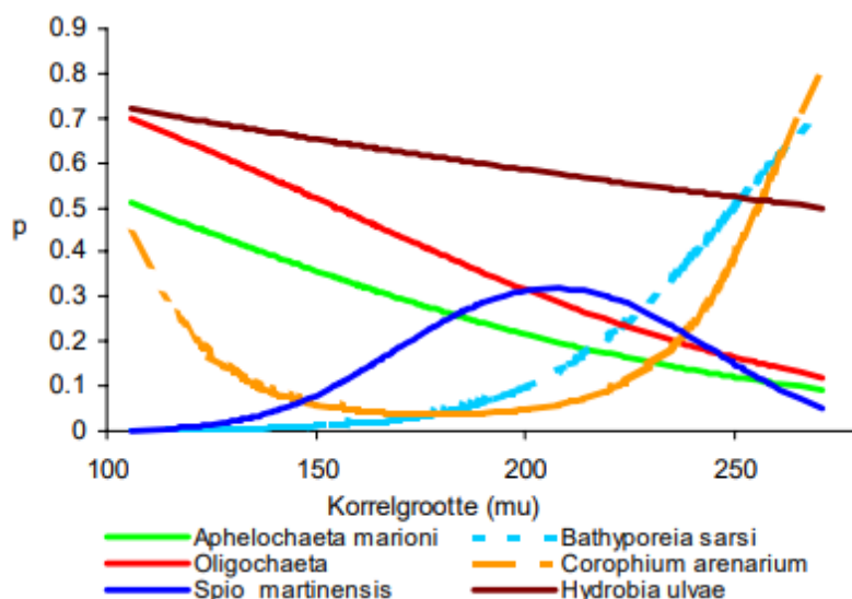
Figuur 3-43- Trefkans voor bodemdieren soorten als functie van de mediane sediment korrelgrootte ( \mu m) berekend door middel van logistische regressie (in Escaravage et al., 2003). Let op bij het maken van dit figuur werden bepaalde soorten anders genoemd dan tegenwoordig: Hydrobia ulvae heet nu Peringia ulvae .
