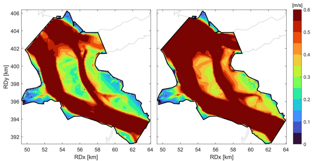
Figuur 3-6. Een ruimtelijk overzicht van de gemiddelde piekstroomsnelheden (links) (de Vet et al., 2017) en de maximale piekstroomsnelheden (rechts) (Ecotopenkaart van 2021). De kleurenschaal loopt van 0 tot 0,6 m/s om de focus te leggen op de stroming op de intergetijdgebieden.
