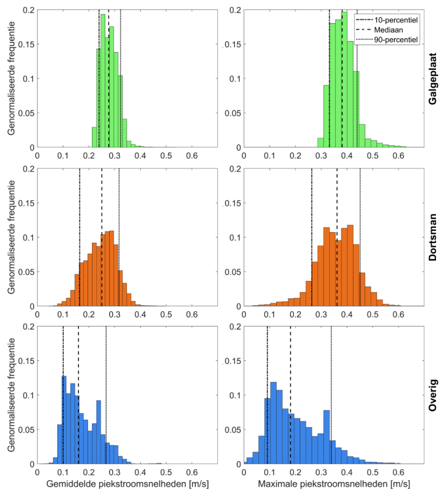
Figuur 3-7. Histogram per deelgebied (zie Figuur 3-15) van de gemiddelde piekstroomsnelheden (De Vet et al., 2017) (links) en de maximale piekstroomsnelheden (Ecotopenkaart van 2021) (rechts). De frequentie van het voorkomen is genormaliseerd door het te delen door het totaal aantal datapunten per reeks. De stroomsnelheden zijn alleen beschouwd voor gebieden die tussen 1990 en 2021 altijd tussen MLW en MHW lagen.
