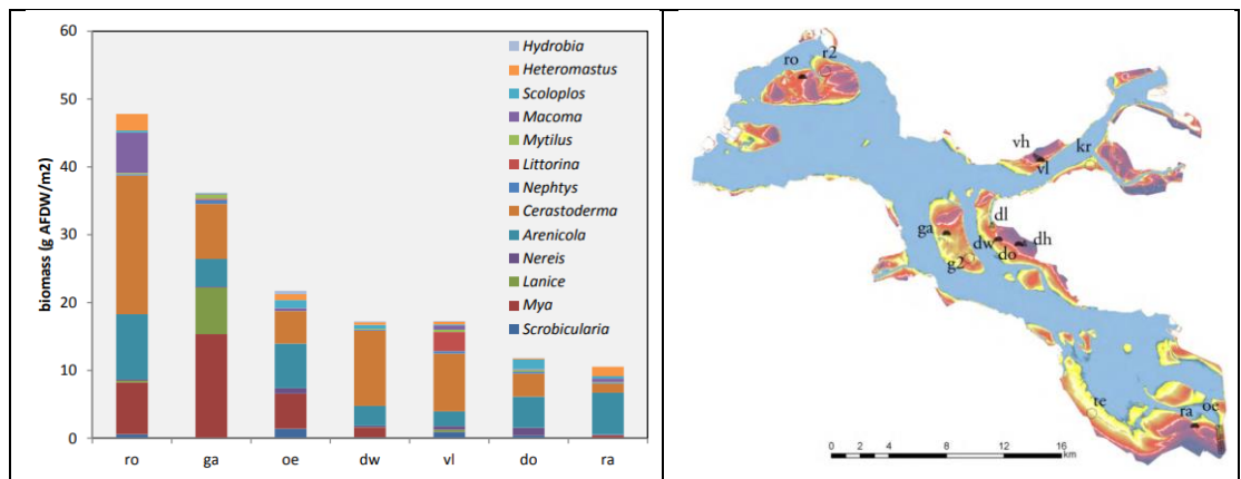
Figuur 3-40. Biomassa (gAFDW/m 2 ) van 13 dominante soorten in zeven gebieden gesorteerd van rijk (Roggenplaat) naar arm (Rattekaai) uit Zwarts et al. (2011). Let op bij het maken van dit figuur werden bepaalde soorten anders genoemd dan tegenwoordig: Hydrobia heet nu Peringia .
