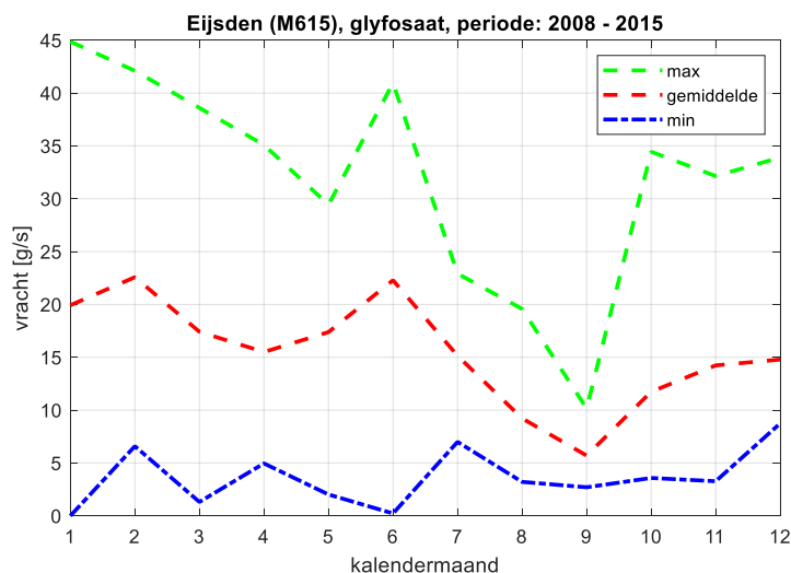
Figuur 4-13 Vrucht glyfosaat bij Eijsden per kalendermaand
