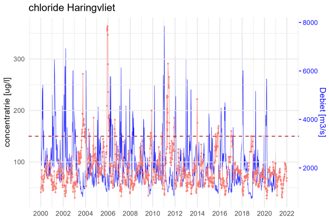
Figuur 7-4: tijdserie van totaal chloride bij Haringvliet met de tijdserie van de afvoer op de secundaire y-as (de rode stippellijn geeft de wettelijke norm 150 µg/l). (voor 2017 = station Scheelhoek, na 2017 = Stad aan 't Haringvliet)
