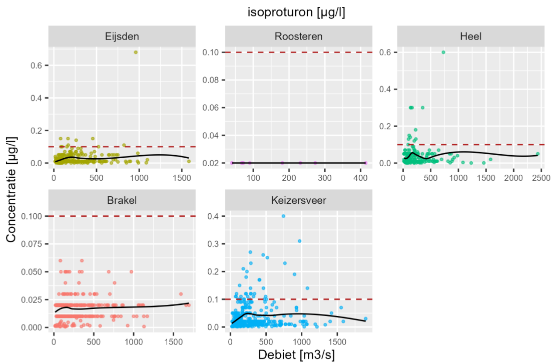
Figuur E-1 Correlatie plot isoproturon voor Maas-locaties met de drinkwater kwaliteitseis (uit de drinkwaterregeling) weergegeven met rode stippellijn (0,1 µg/l). Bij Eijsden, Roosteren en Heel is het debiet bij Eijsden gebruikt, voor Brakel en Keizersveer het debiet bij Keizersveer.
