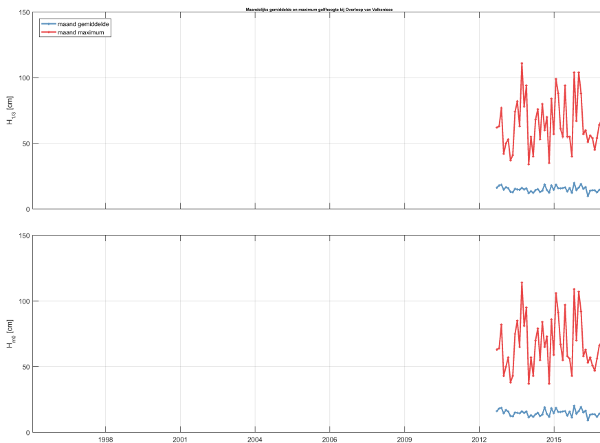
Figuur 2.38: Maandlijks gemiddelde en maximum van de significante golfhoogte H_{1/3} (boven) en H_{m0} (onder) voor station Overloop van Valkenisse.
