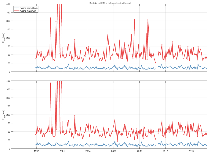
Figuur 2.37: Maandlijks gemiddelde en maximum van de significante golfhoogte H_{1/3} (boven) en H_{m0} (onder) voor station Hansweert.
