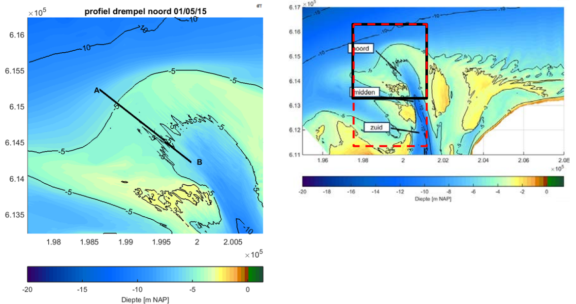
Figuur 3.1 Gebied met multibeam-metingen ter plaatse van verdieping.
