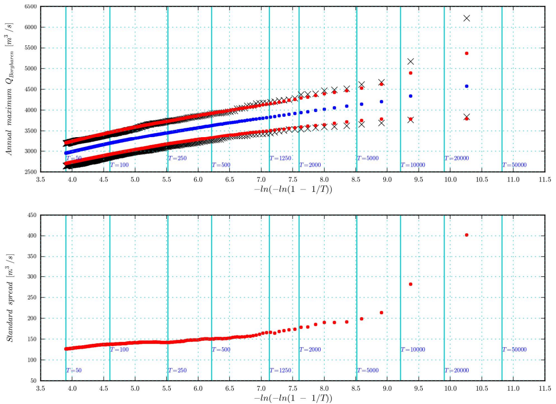
Figuur 4.1 Verloop van het standaard gemiddelde en standaard spreiding van de per empirische herhalingsijd T_n met GRADE berekende 24x5 jaarmaxima
