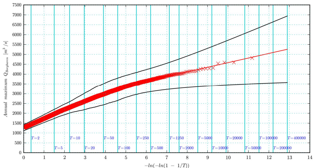
Figure A.1 Afvoer-frequentie lijn en onzekerheidsband voor de Maas bij Borgharen voor een Weissman drempel T_w=100 jaar voor de onzekerheidsbanden
