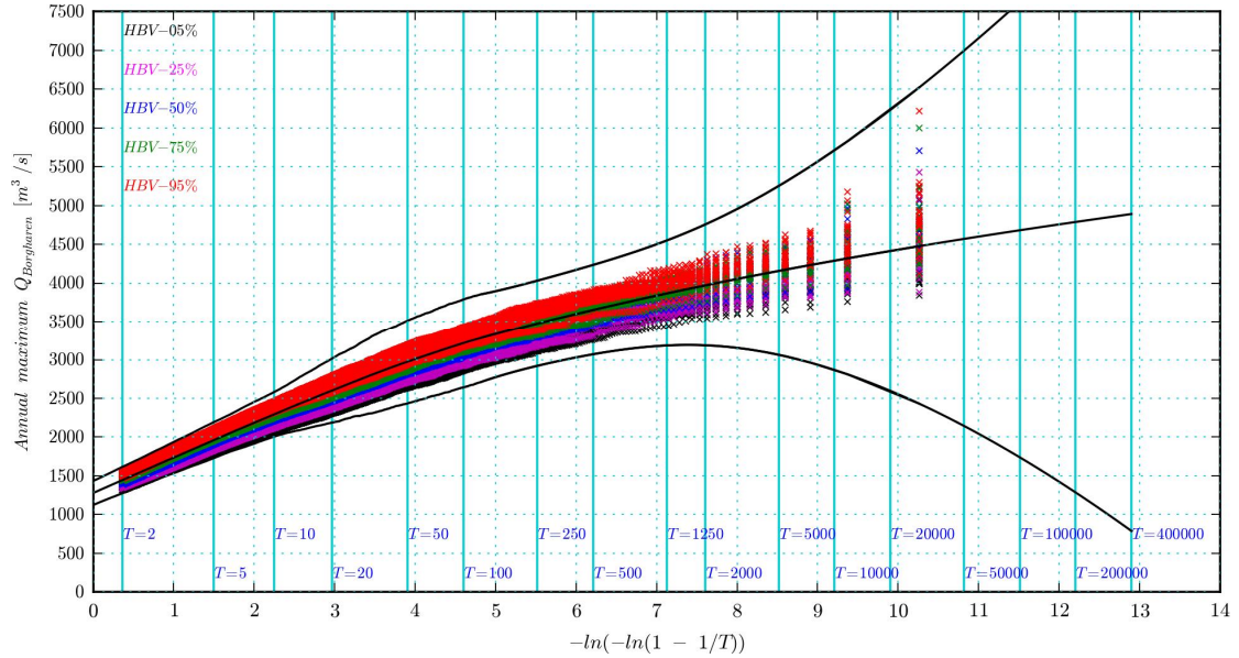
Figuur 3.2 Frequentielijn en onzekerheidsband voor jaarmaxima van de Maas. Hier met een T_W = 125 jaar en een GPD verdeling in de Weissman procedure
