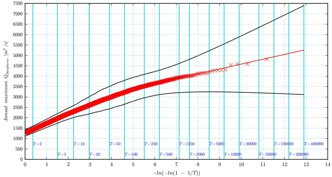
Figure A.3 Afvoer-frequentie lijn en onzekerheidsband voor de Maas bij Borgharen voor een Weissman drempel T_w=250 jaar voor de onzekerheidsbanden
