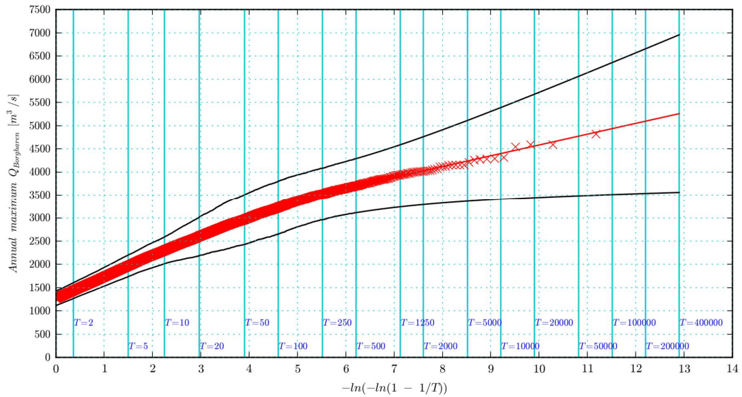
Figure A.2 Afvoer-frequentie lijn en onzekerheidsband voor de Maas bij Borgharen voor een Weissman drempel T_w=125 jaar voor de onzekerheidsbanden
