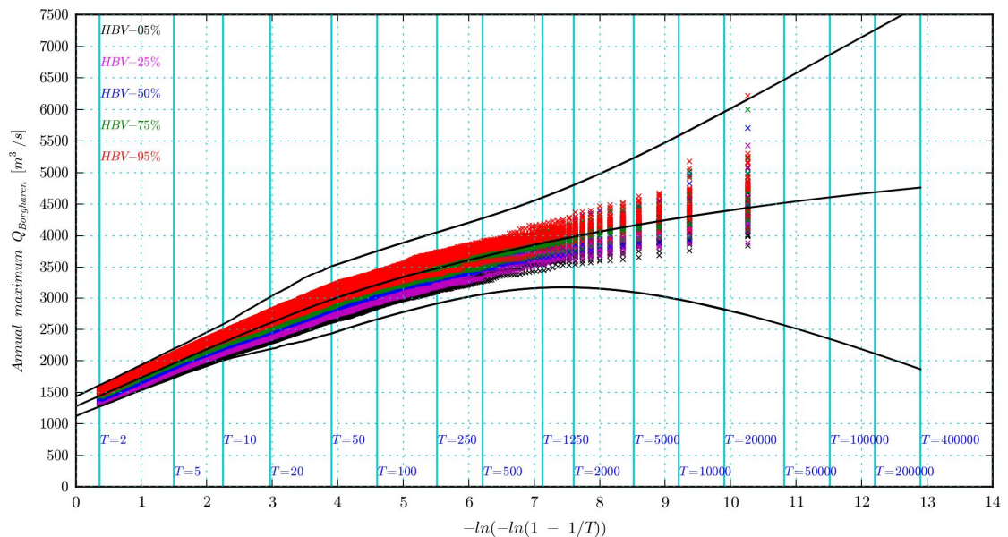
Figuur 3.3 Frequentielijn en onzekerheidsband voor jaarmaxima van de Maas. Hier met een T_W = 50 jaar en een GPD verdeling in de Weissman procedure
