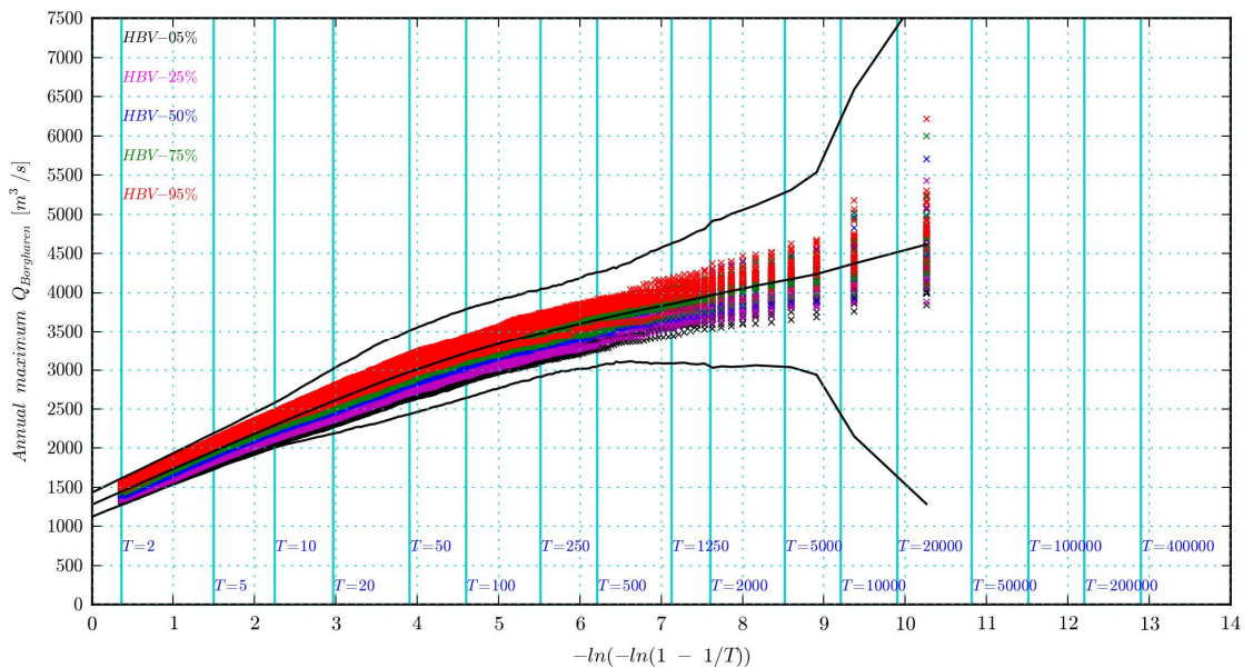
Figuur 4.2 Resultaat van de GRADE onzekerheidsanalyse voor de Maas als hierbij geen Weissman procedure voor smoothing en extrapolatie van de staart wordt toegepast
