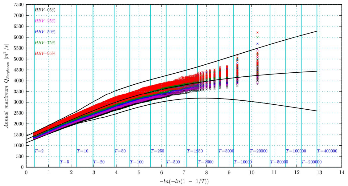
Figuur 4.3 Frequentielijn en onzekerheidsband voor jaarmaxima van de Maas. Hier met een T_W = 50 jaar en een GPD verdeling in de Weissman procedure, en het uitsluiten van de datapunten voorbij een herhalings-tijd van 10000 jaar
