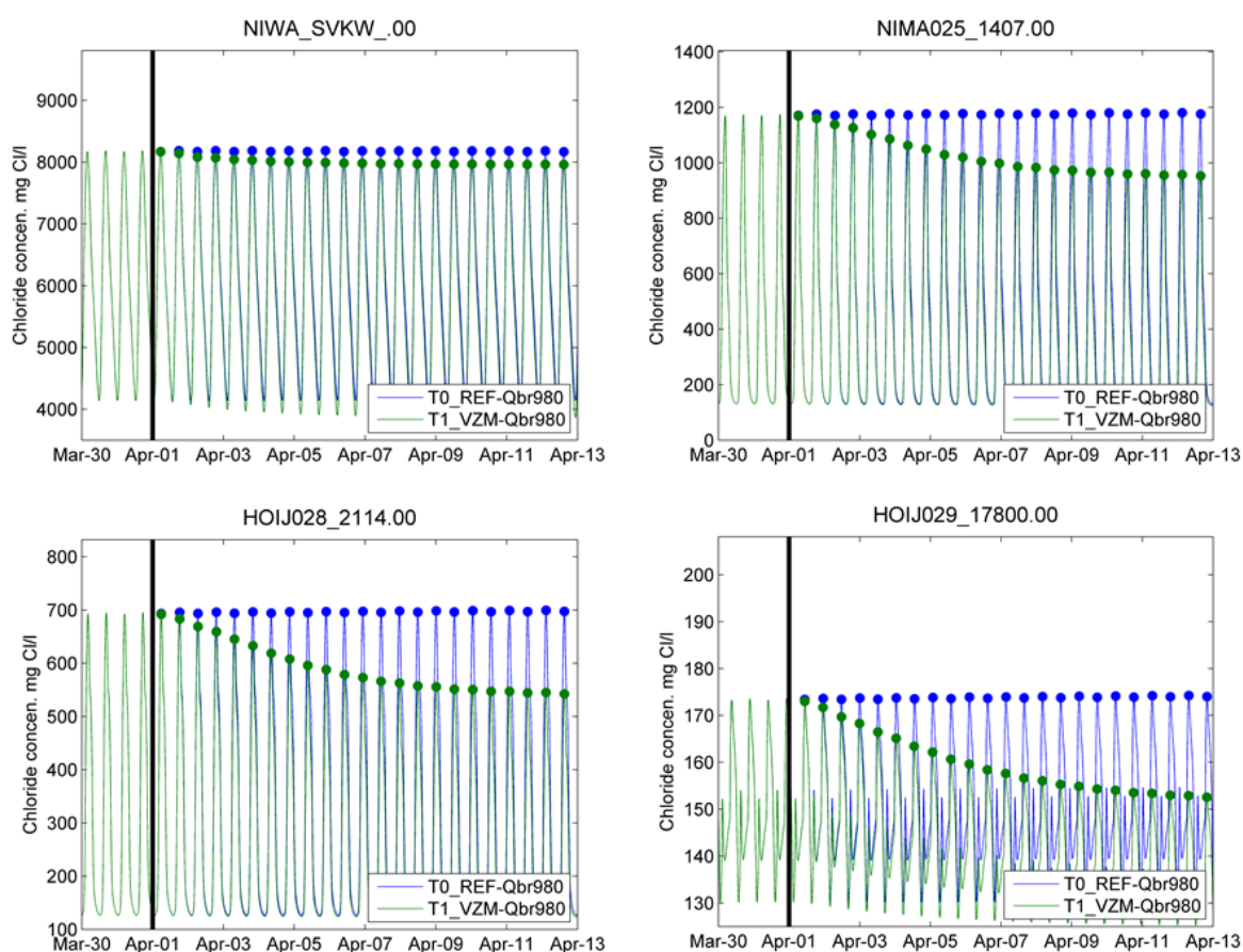
Figuur 5.4 Ontwikkeling zoutconcentraties voor de referentie situatie (T0) en voor wanneer de onttrekking richting het Volkerak-Zoommeer wordt stopgezet: 50 \text{ m}^3/\text{s} \rightarrow 0 \text{ m}^3/\text{s} (T1). De schaal van de verticale as is verschillend voor de 4 figuren
