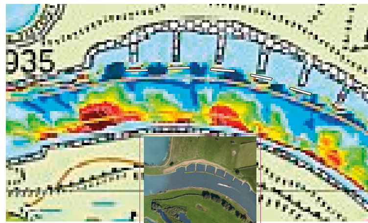
Figuur 3.8 Pilottraject Zutphen km 934 – km 935
