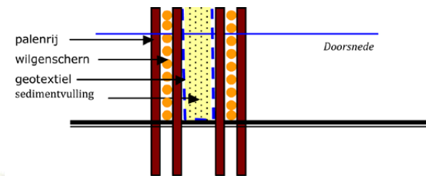
Figuur 2.3 Voorbeeld van een palenrij die een kribvak nabij Ewijk gedeeltelijk afsluit
