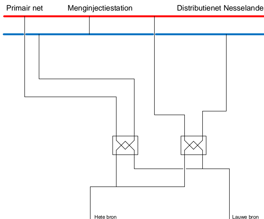
Figuur 3-2: Inpassing HTO Rotterdam-Nesselande zonder warmtepomp met enkele warmtewisselaars. Er zijn ook varianten uitgewerkt met dubbele warmtewisselaars.
