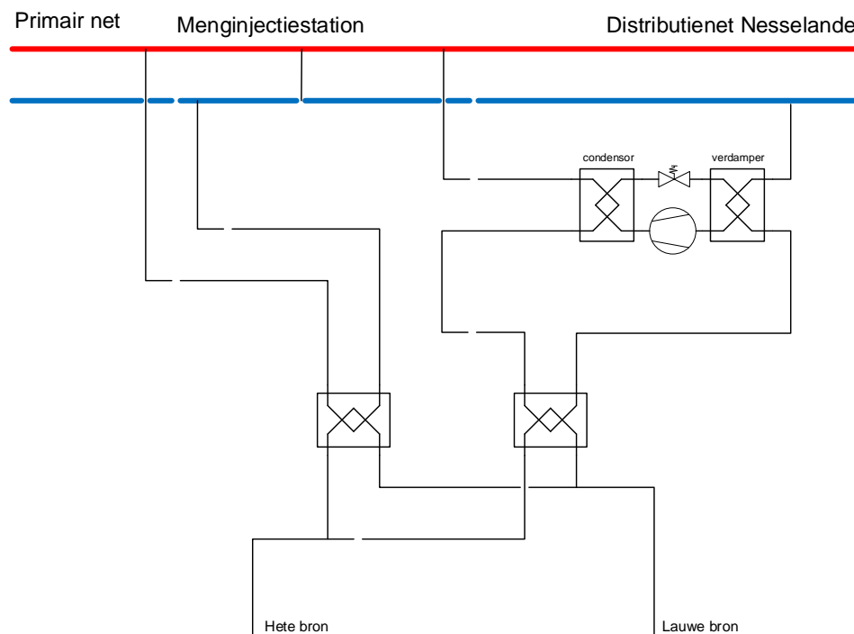
Figuur 3-3: Inpassing HTO Rotterdam-Nesseland met warmtepomp met enkele warmtewisselaars. Er zijn ook varianten uitgewerkt met dubbele warmtewisselaars.
