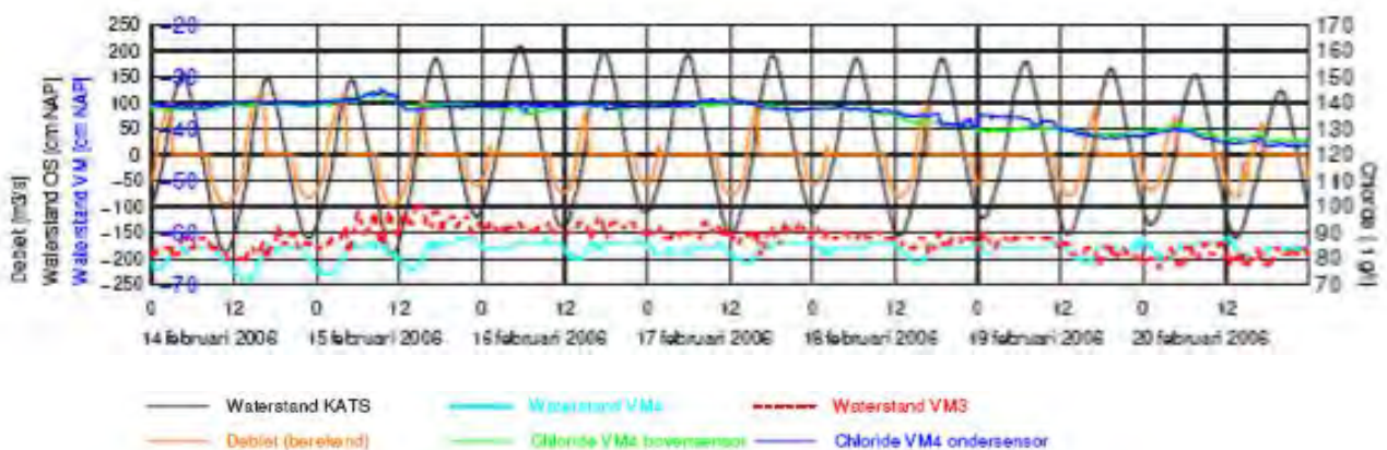
Figuur 2.6 Chloridemetingen (in 0.1 g/l) voor de periode 14 tot en met 20 februari voor meetpaal VM4 (pers.com. P. Lieveense, RWS Directie Zeeland)
